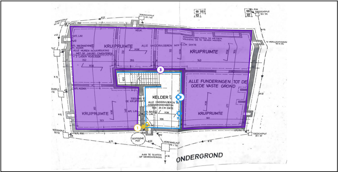
Legende van plan 1.1: Funderingsplan
