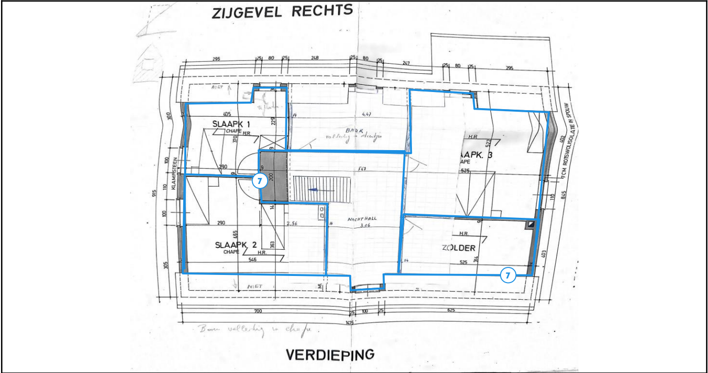
Legende van plan 1.6: Grondplan verdieping
