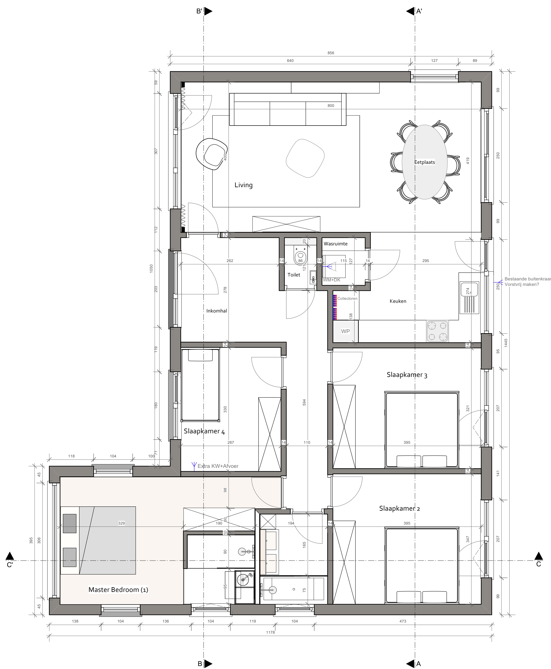
GRONDPLAN NIEUWE TOESTAND - SCHAAAL 1:50
