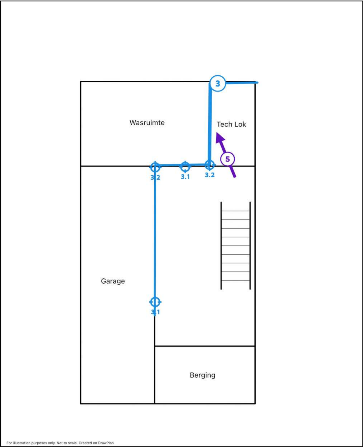
Legende van plan 1.2: Garage en kelder
