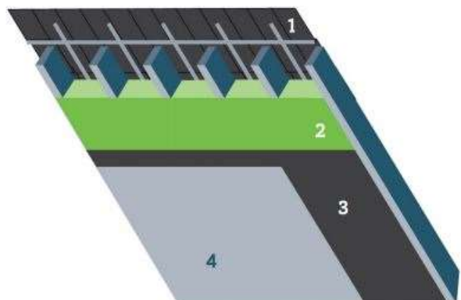
1. Onderdak | 2. Isolatie | 3. Dampscherm | 4. binnenaafwerking
