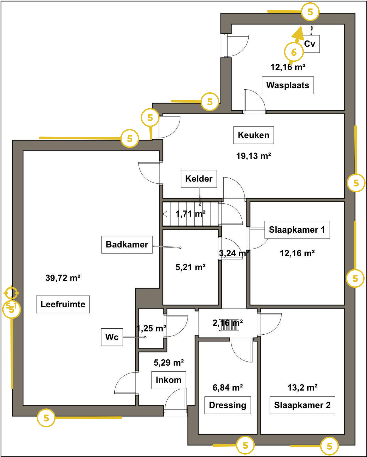
Legende van plan 1.6: Gelijkvloers .3
