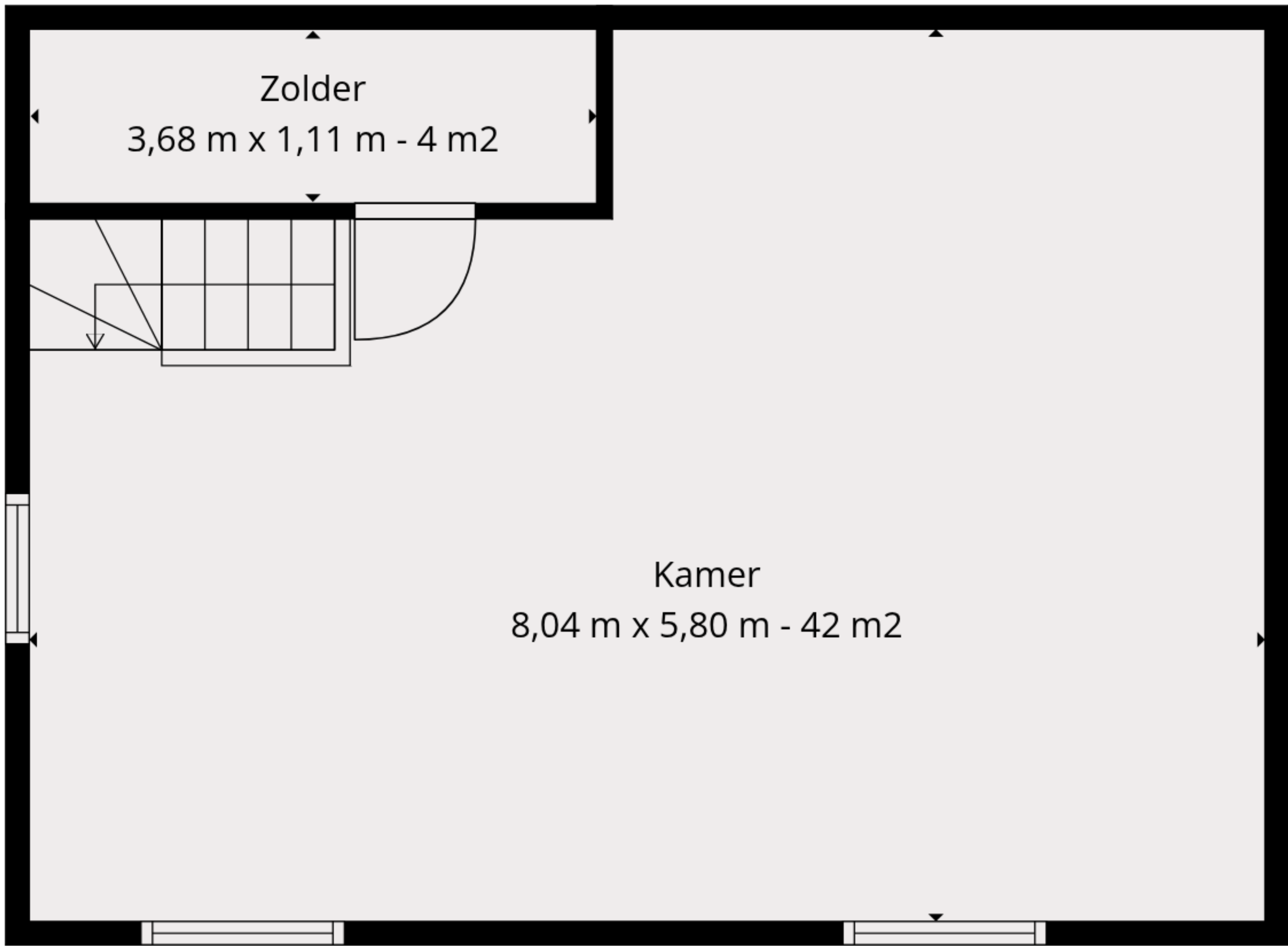
2e Verdieping
