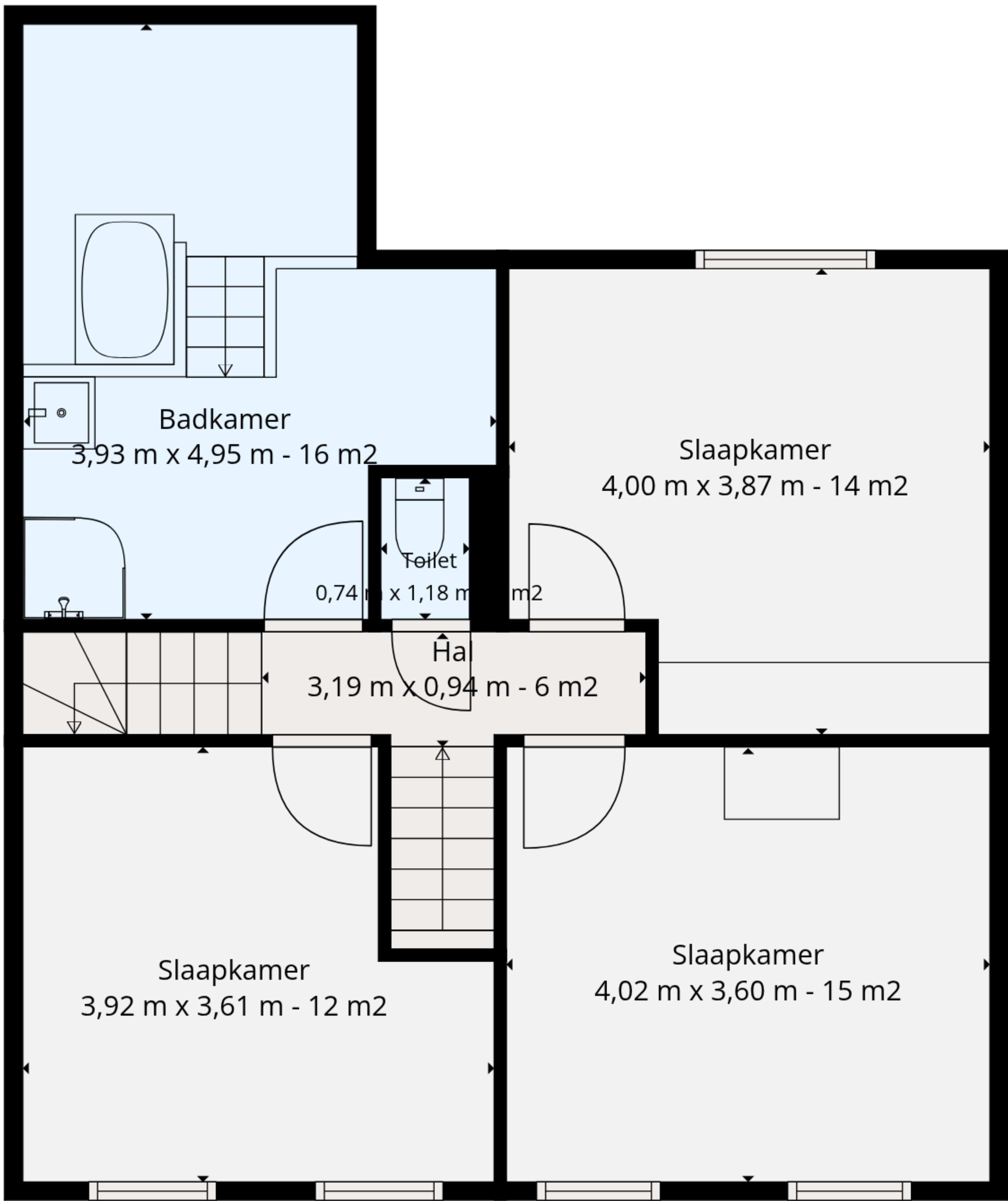
1e Verdieping
