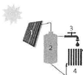
1. Zonnecollector | 2. Opslagvat zonneboiler | 3. Sanitair warm water | 4. Radiator voor ruimteverwarming 5. Opslagvat
