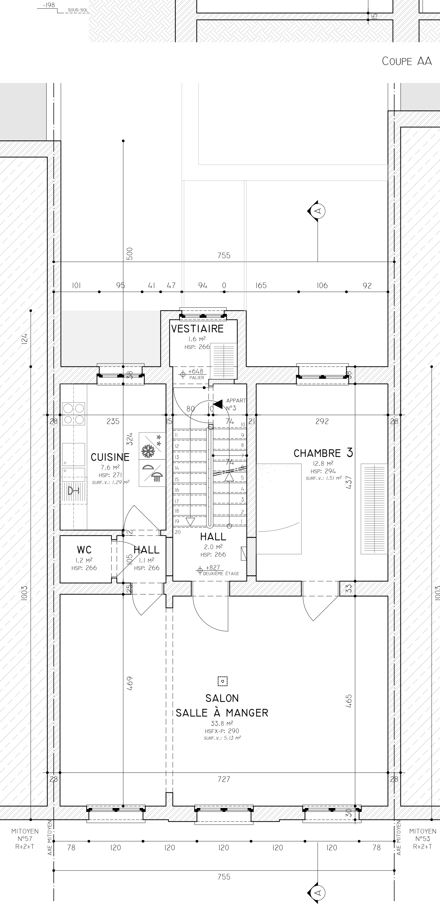
PLAN DU DEUXIÈME ETAGE
