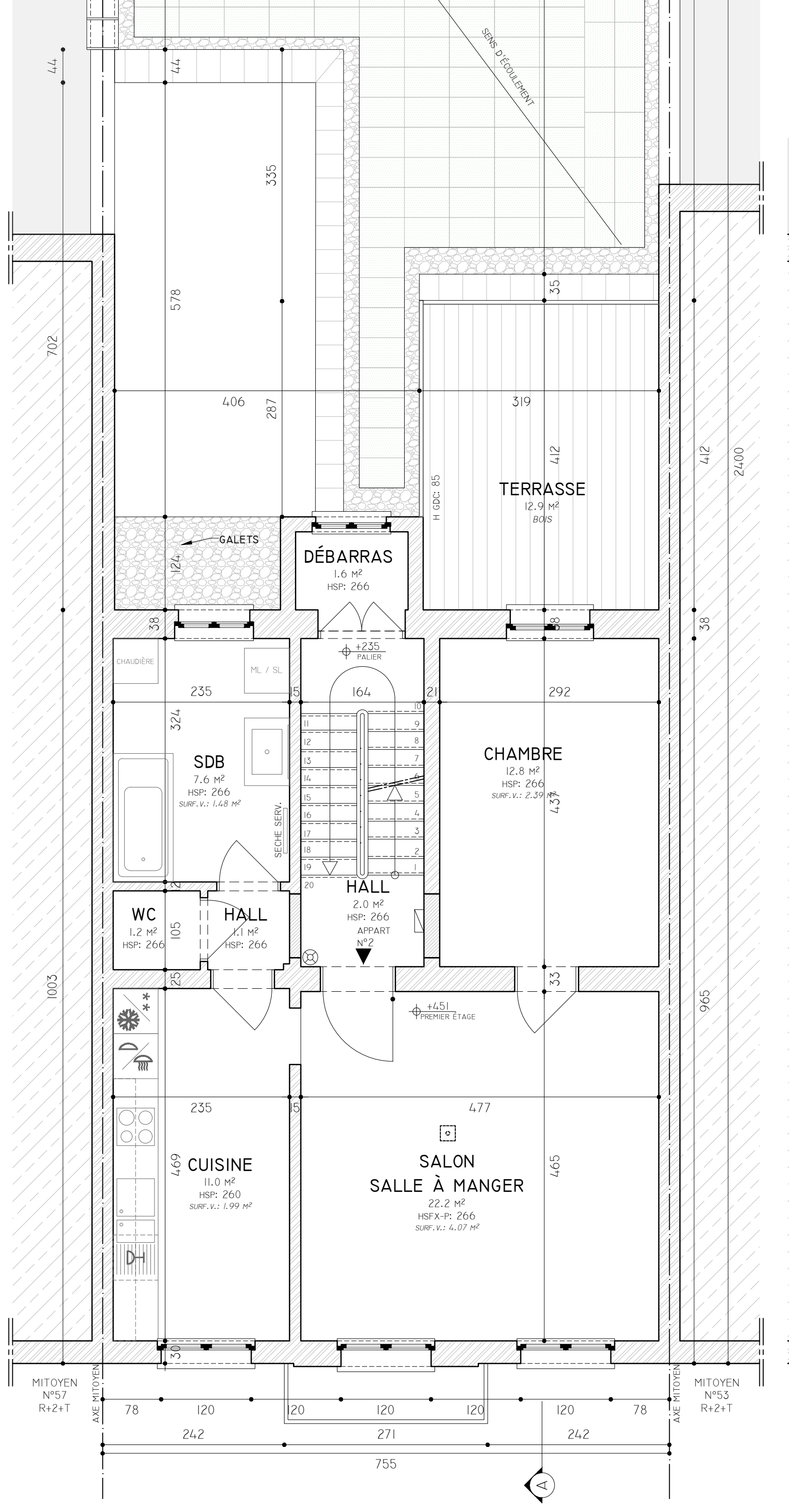
PLAN DU PREMIER ETAGE
