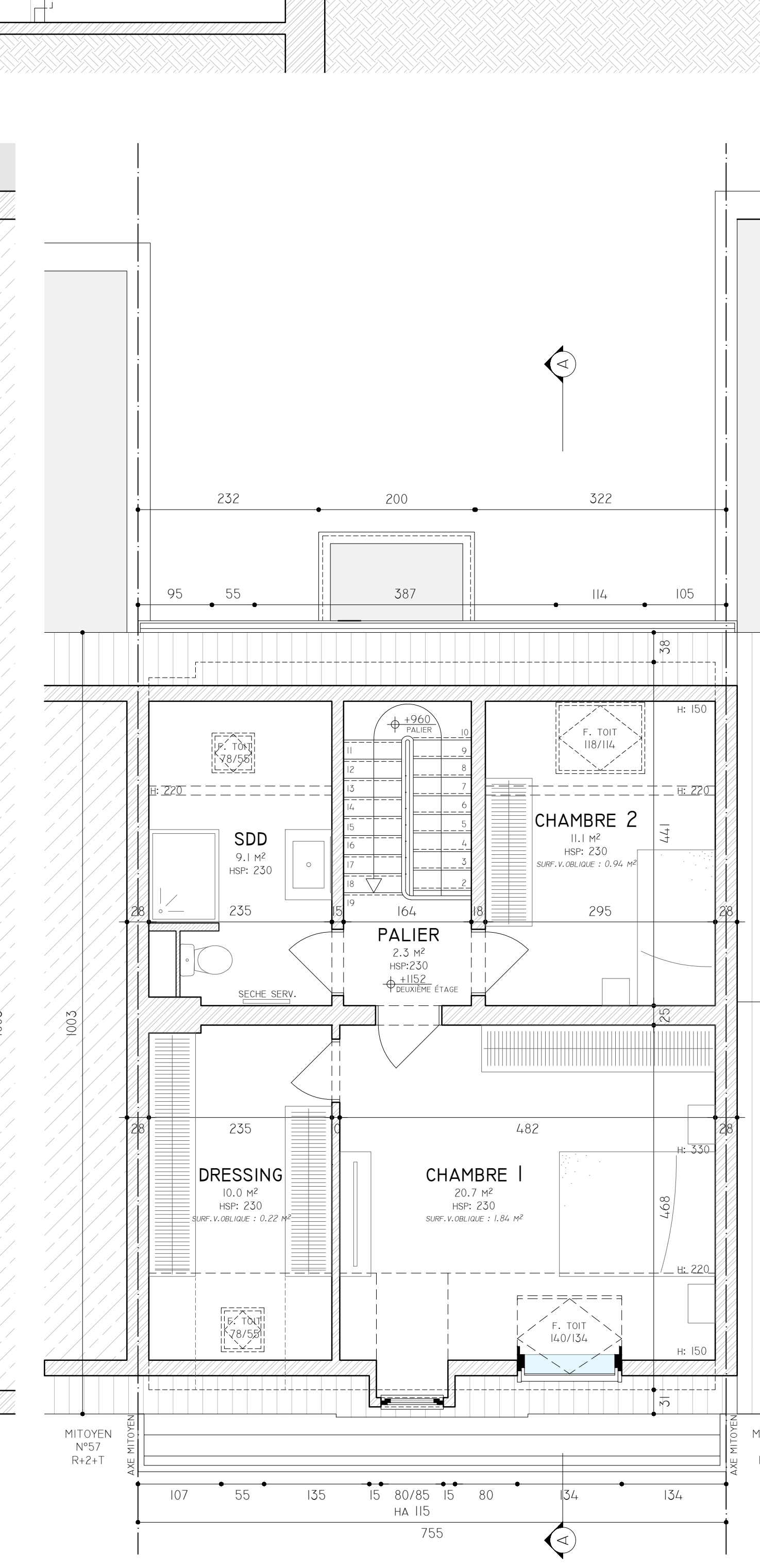
PLAN DES COMBLES
