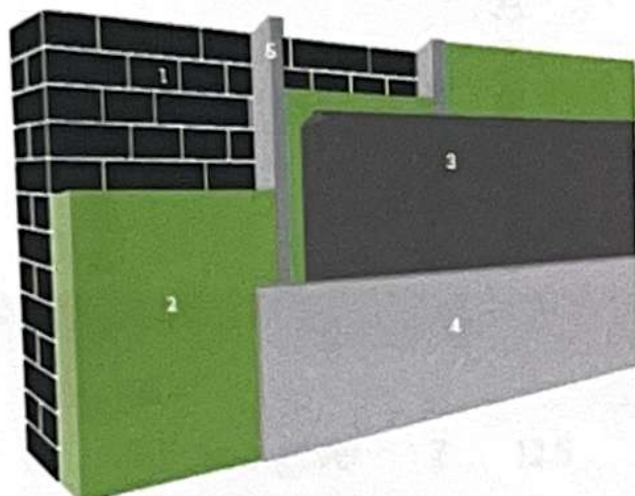
1. Buitenmuur | 2. Isolatie | 3. Vochtscherm | 4. Afwerkingslaag | 5. Stijl- en regelwerk (optioneel)
