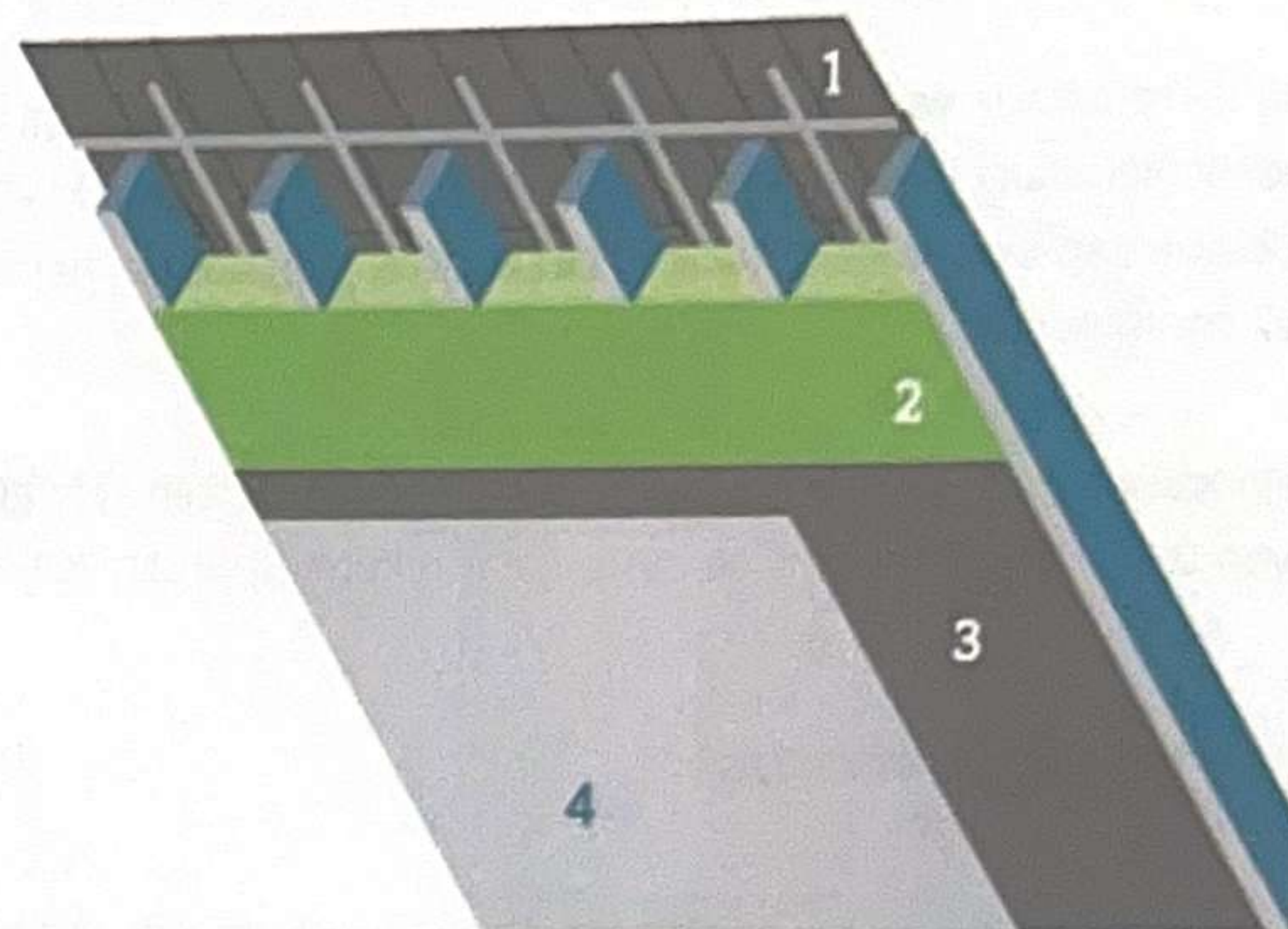
1. Onderdak | 2. Isolatie | 3. Dampscherm | 4. binnenafwerking
