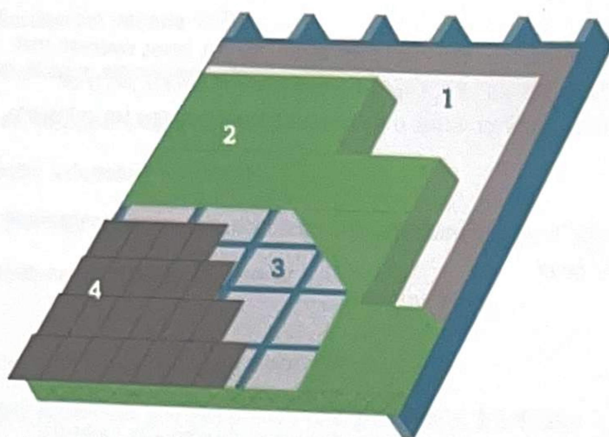
1. Dampscherm | 2. Isolatie | 3. Onderdak | 4. Dakbekleding
