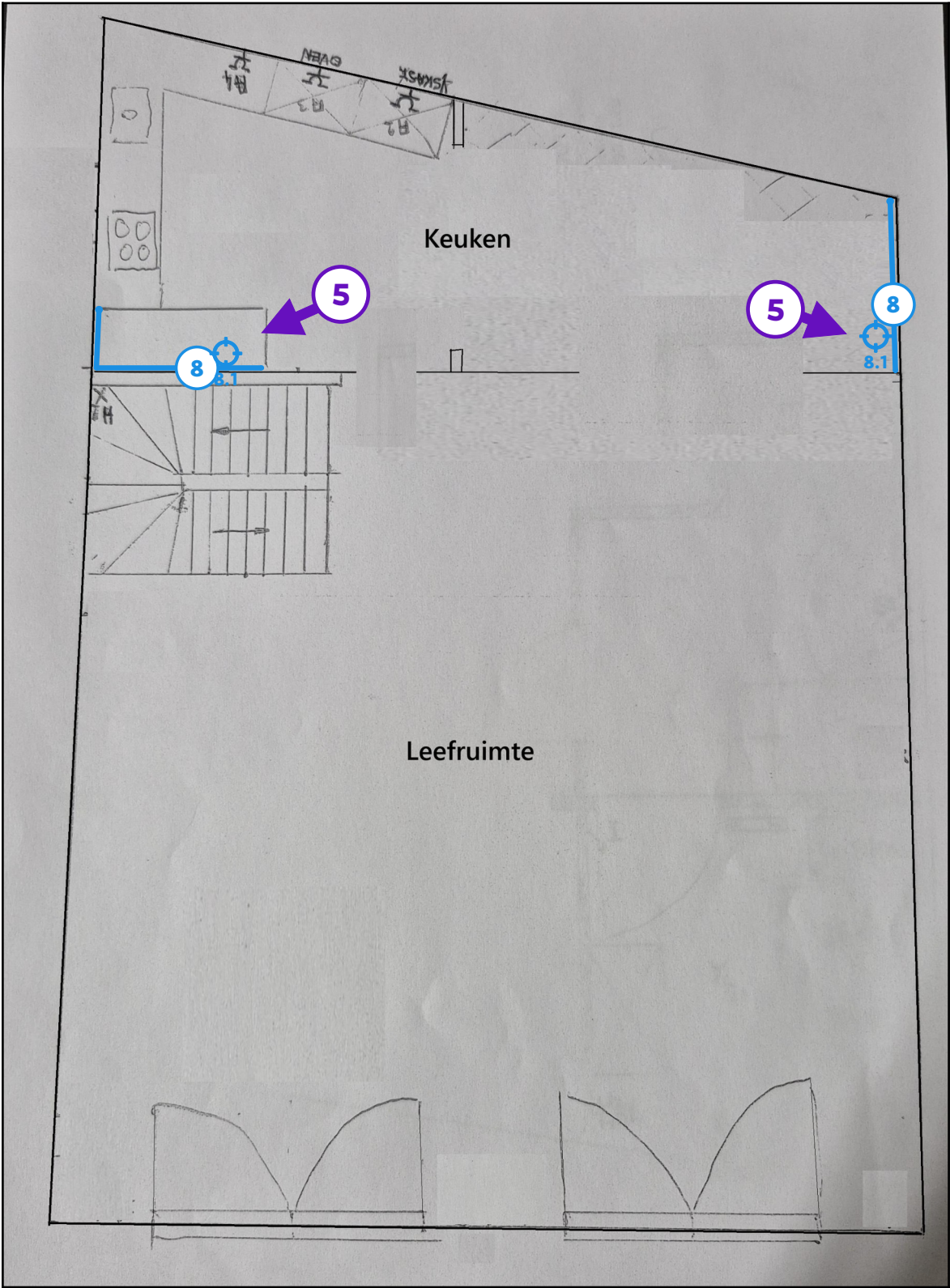
Legende van plan 1.4: Plan 1e verdieping
