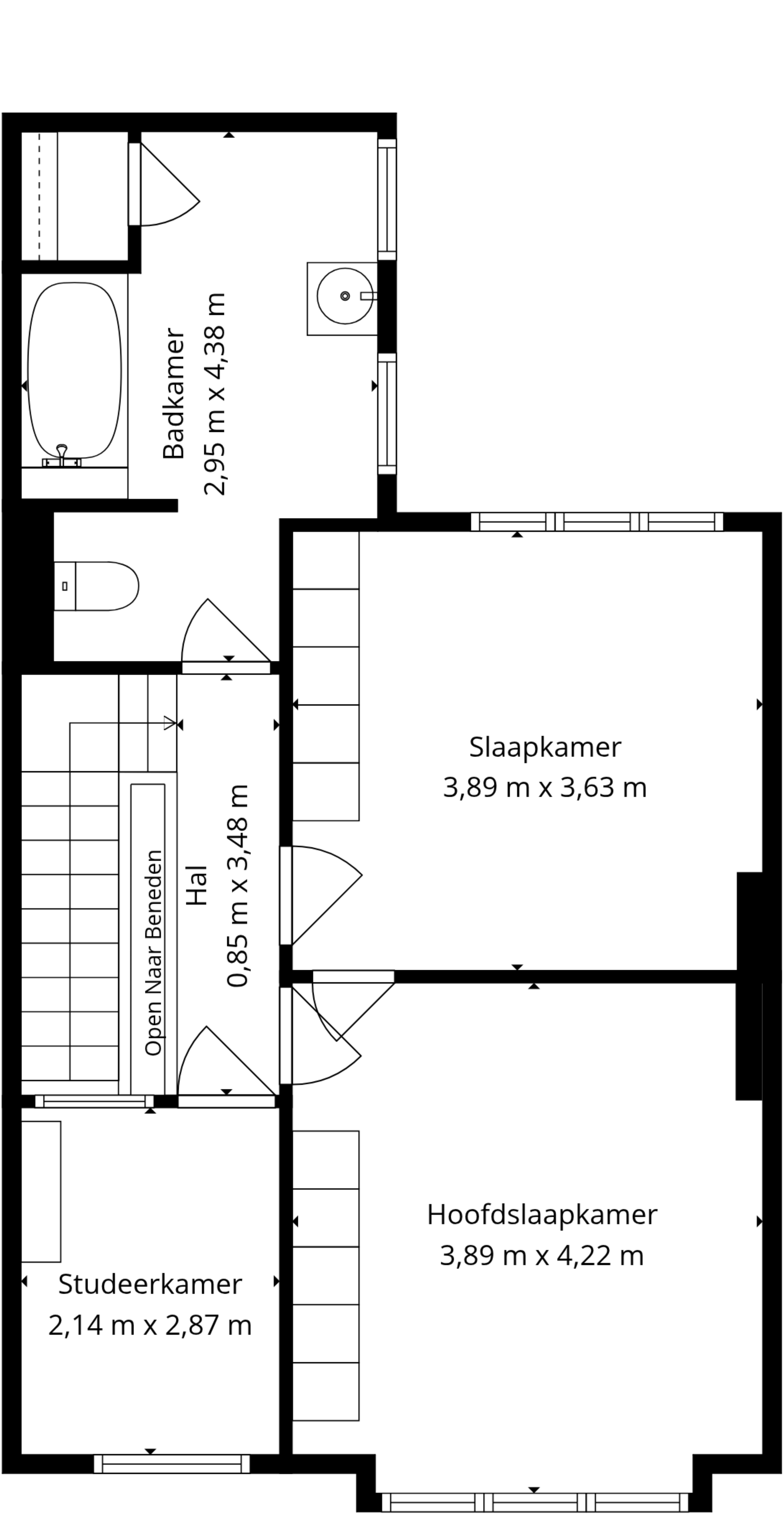
2e Verdieping
