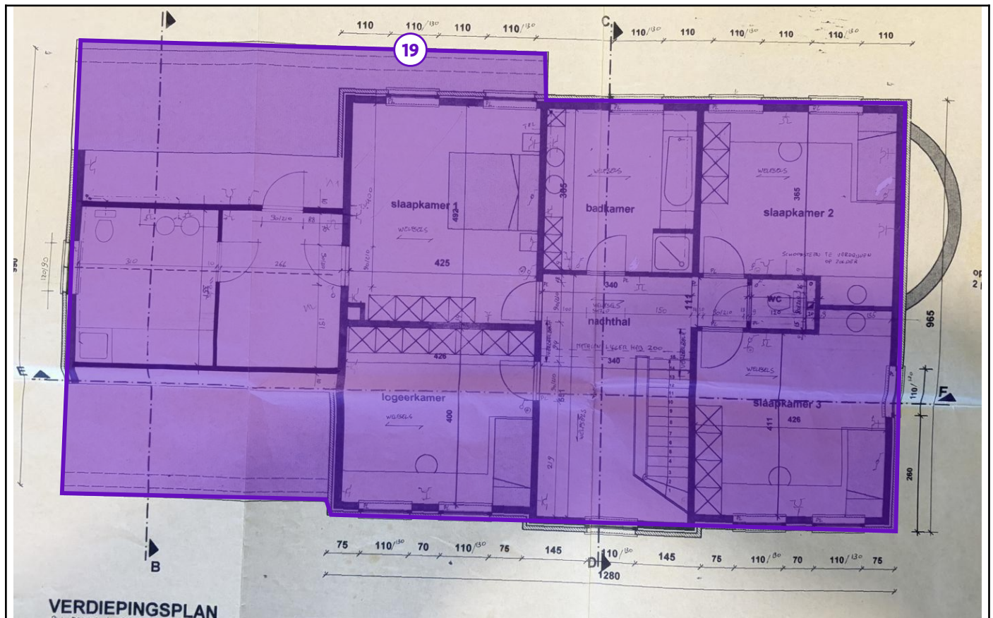
Legende van plan 1.7: Verdiepingplan aanduiding onderdak
