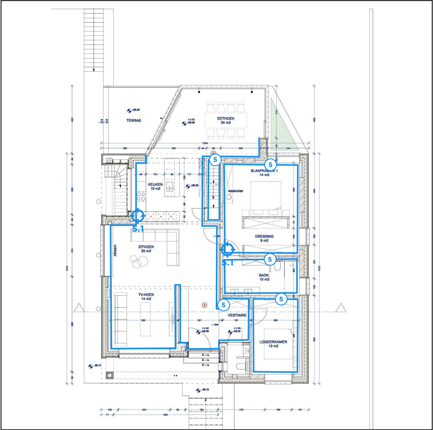
Legende van plan 1.2: gelijkvloers
