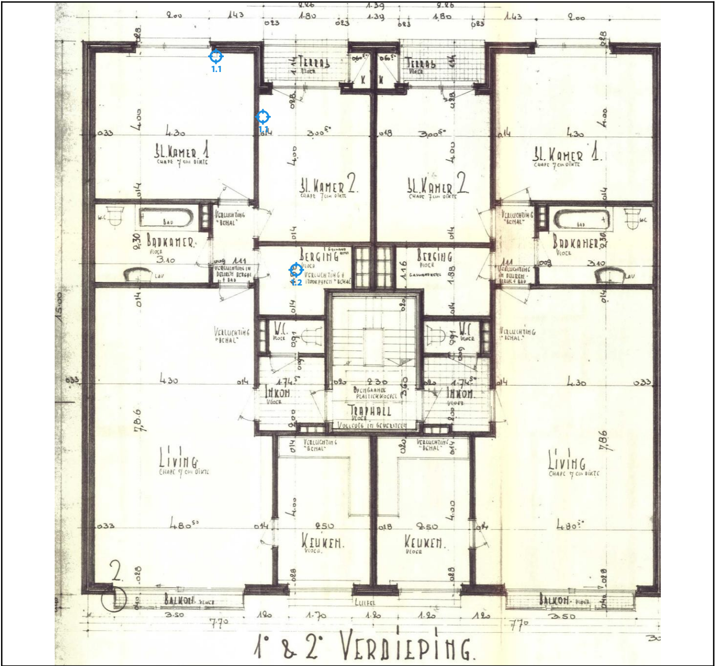
Legende van plan 1.1: Verdiep 2
