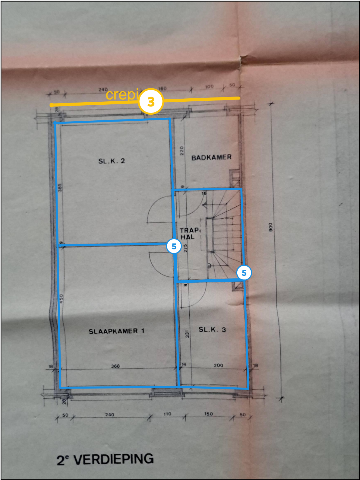
Legende van plan 1.5: 2e verdieping - bezetting muren
