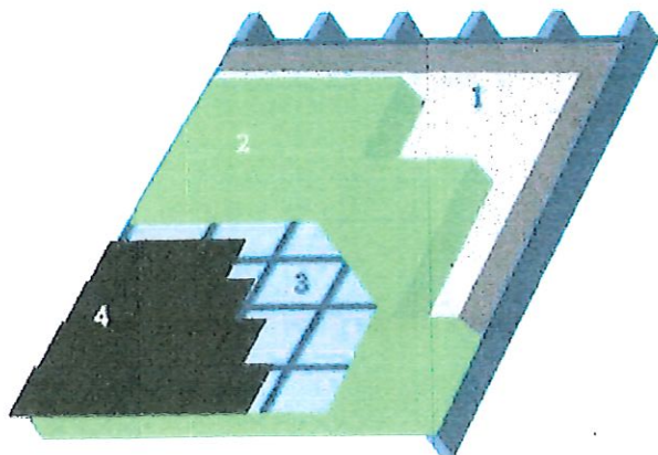
1. Dampschermbaan | 2. Isolatie | 3. Onderdak | 4. Dakbedekking
