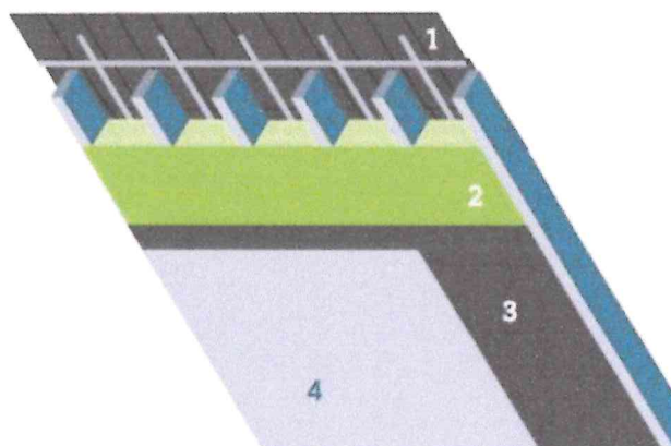
1. Onderdak | 2. Isolatatie | 3. Dampscherm | 4. binnenafwerking
