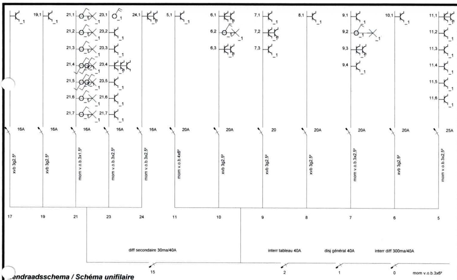
Enddraadsschema / Schéma unifilaire
