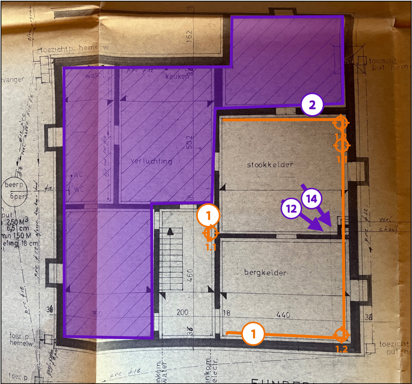
Legende van plan 1.7: Kelder + kruipruimte
