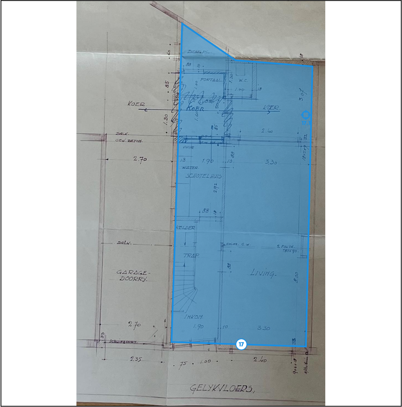
Legende van plan 1.7: plan - gelijkvloers
