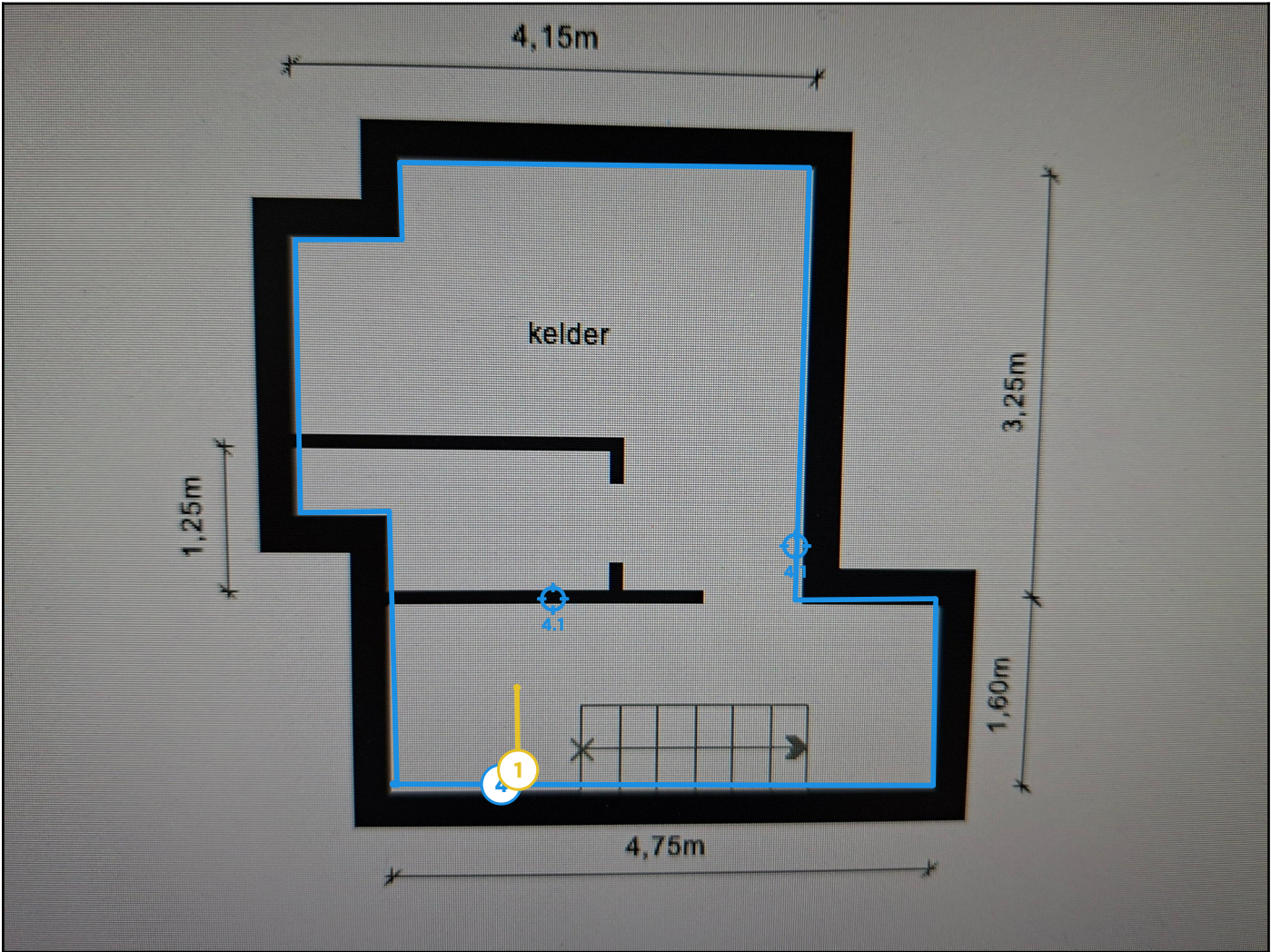
Legende van plan 1.1: Grondplan kelder
