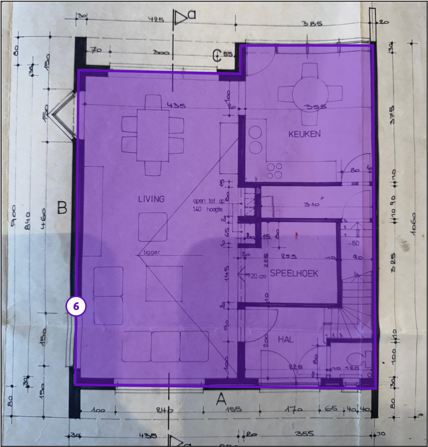
Legende van plan 1.1: Verdieping V0
