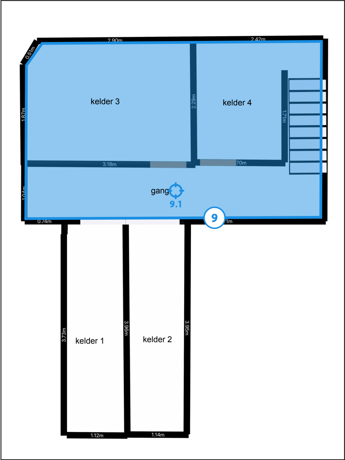
Legende van plan 1.2: Kelder (plafonds)
