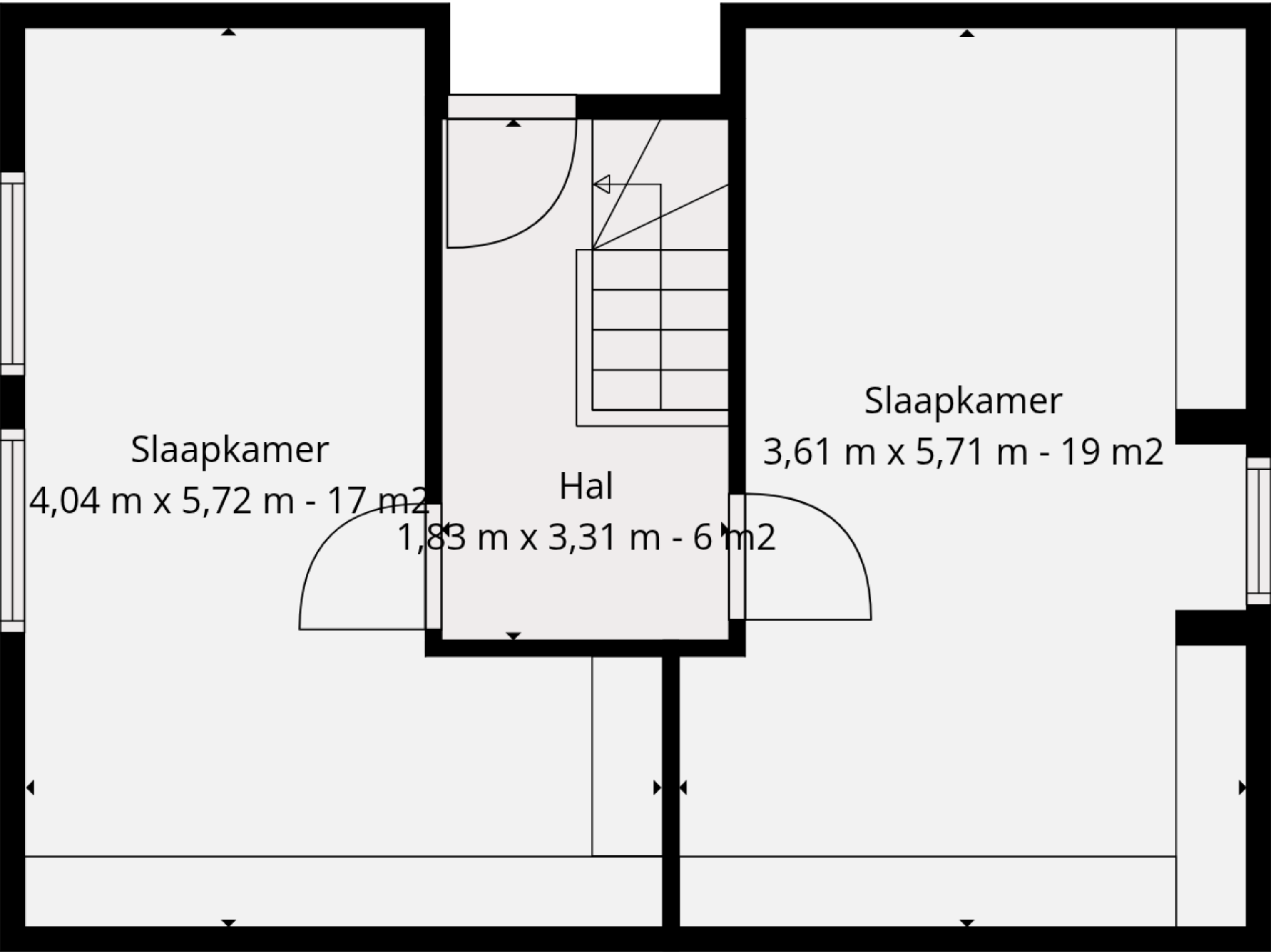
2e Verdieping
