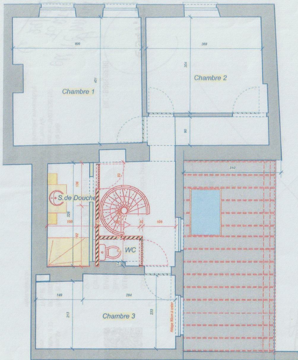
PD3 21/06/2025 Plan étage PROJETÉ
