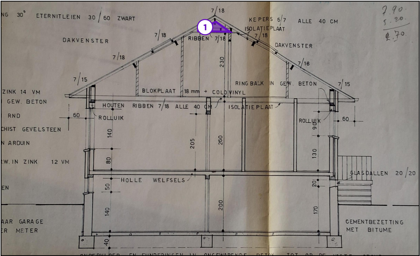
Legende van plan 1.8: Doorsnede
