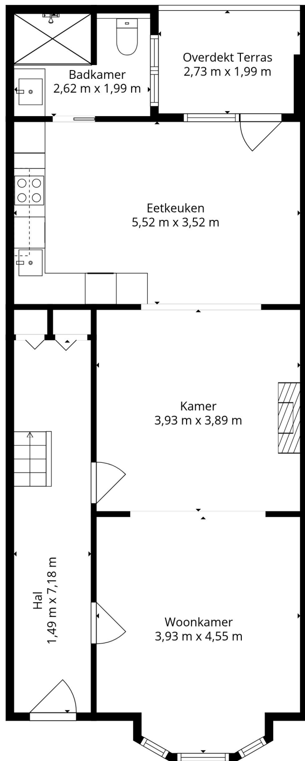
1e Verdieping
