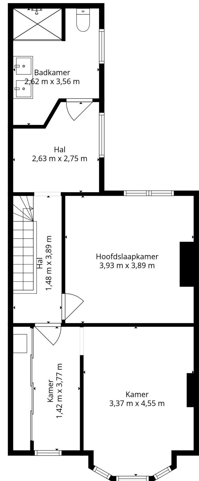
3e Verdieping
