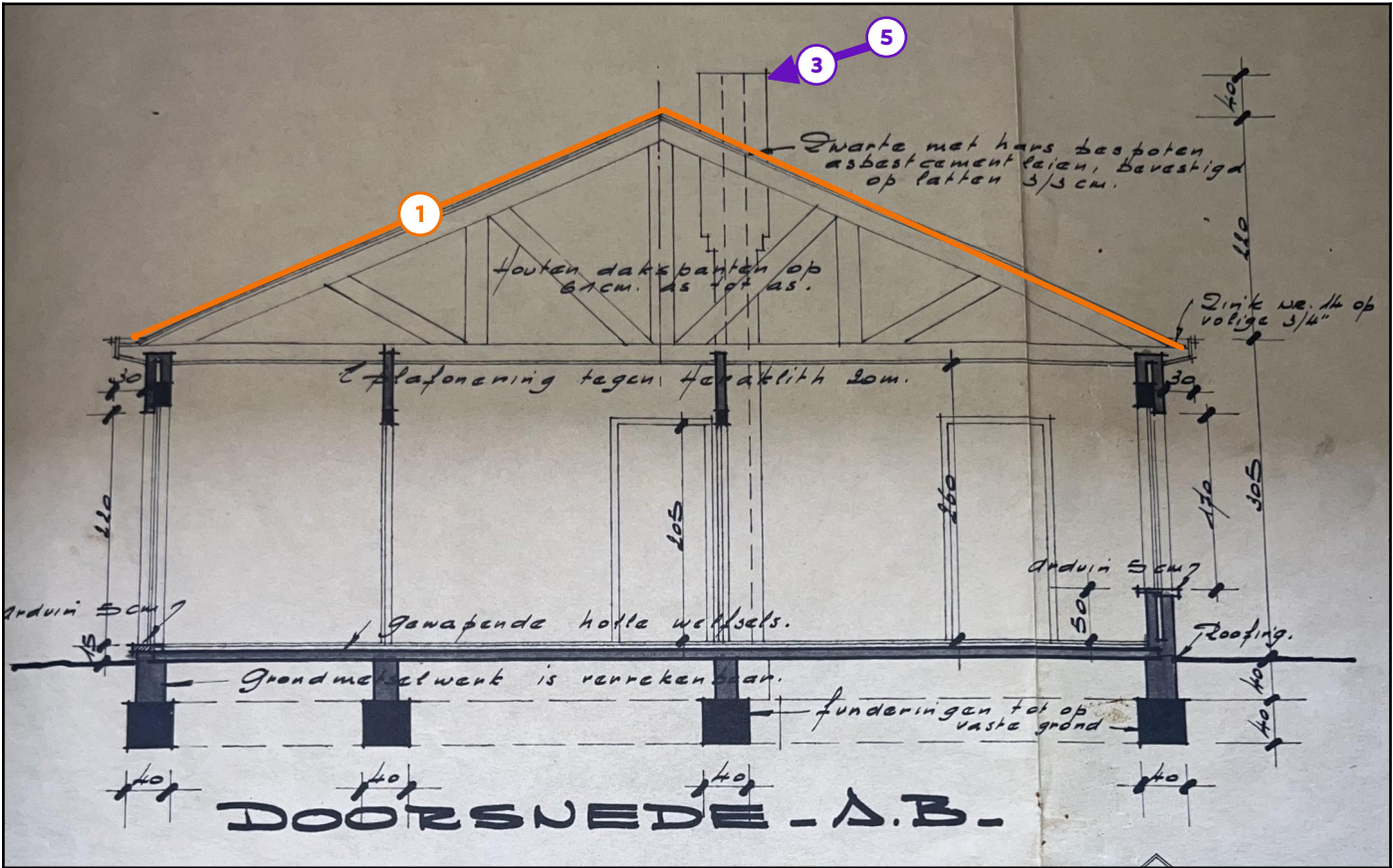
Legende van plan 1.4: Snede
