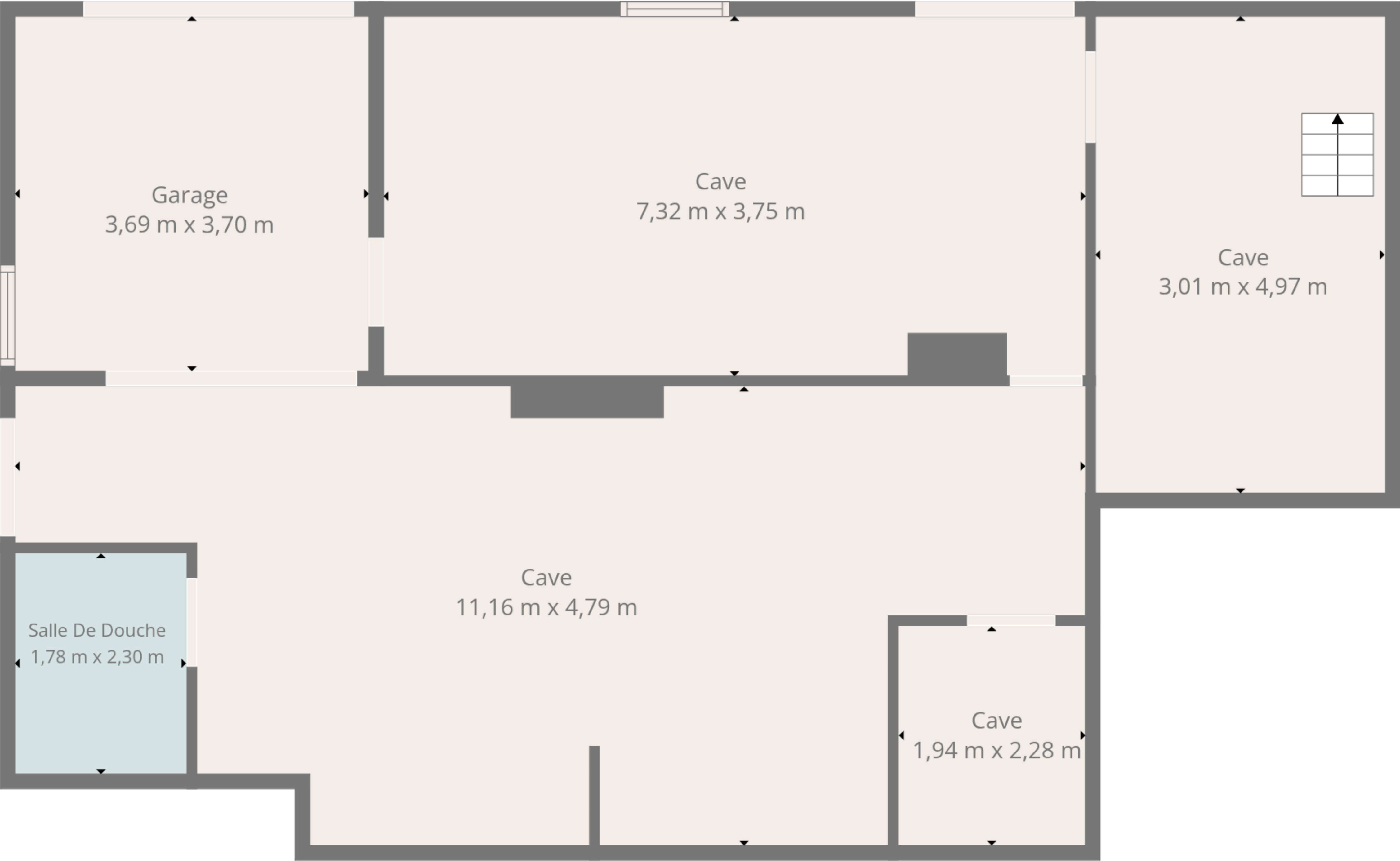
Sous-sol
