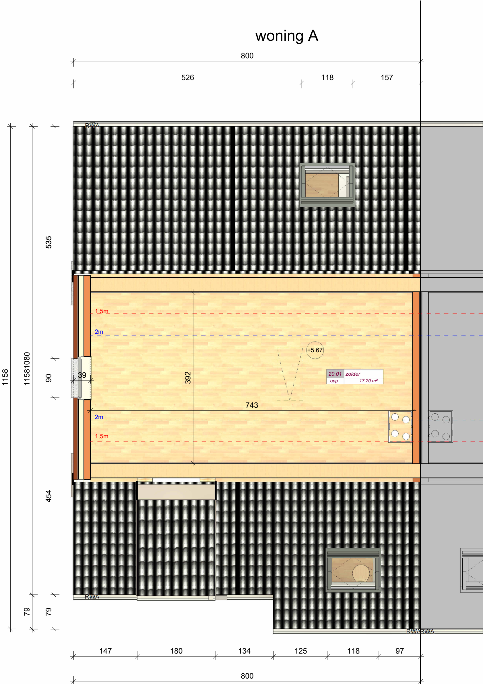
1 woning A zolder 1 : 50
