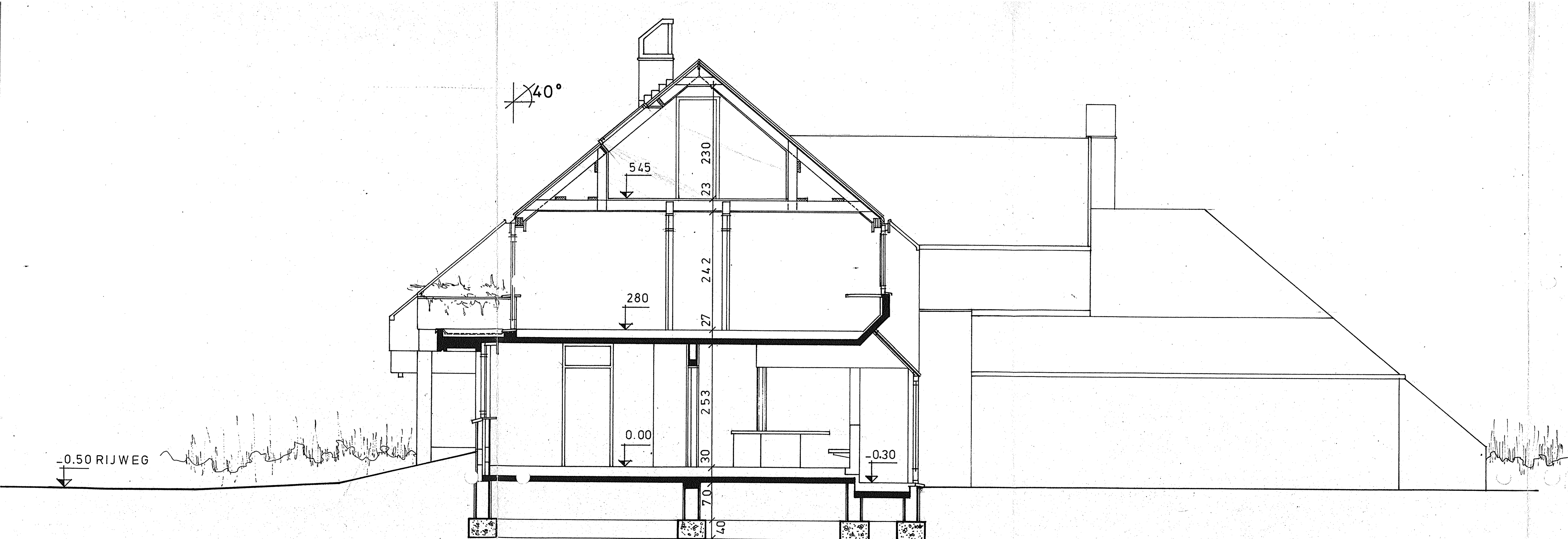
DOORSNEDE AB fundering tot op draagvaste grond
