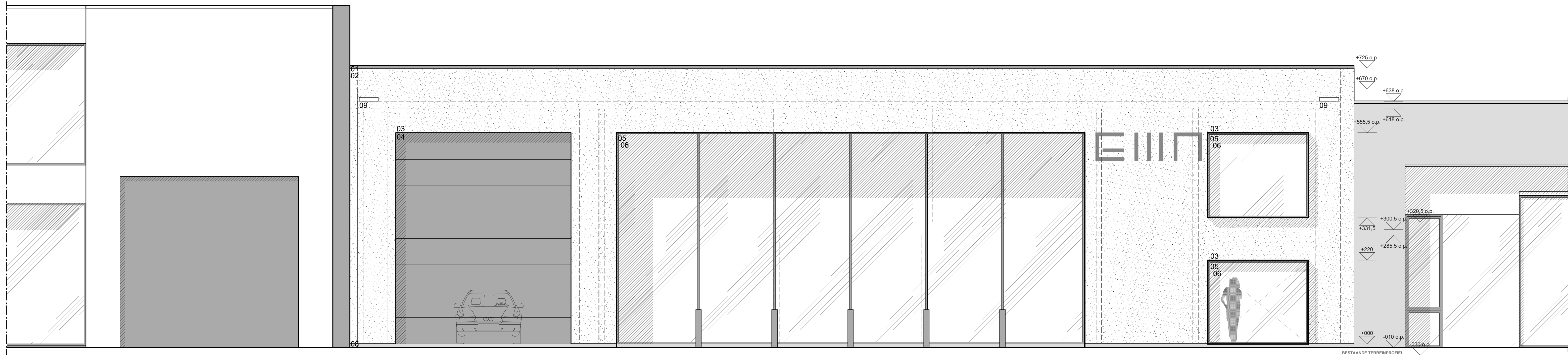
VOORGEVEL VARIANT - NT SCHAAL 1/50
