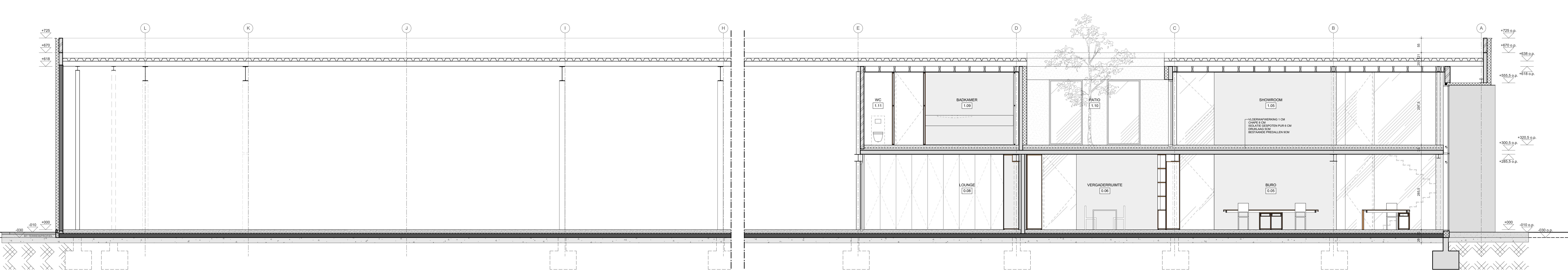
SNEDE AA - NT SCHAAL 1/50
