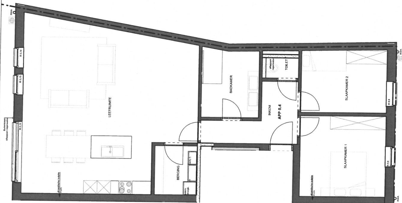
APPARTEMENT 0.4 SCHAAL: 1:100
