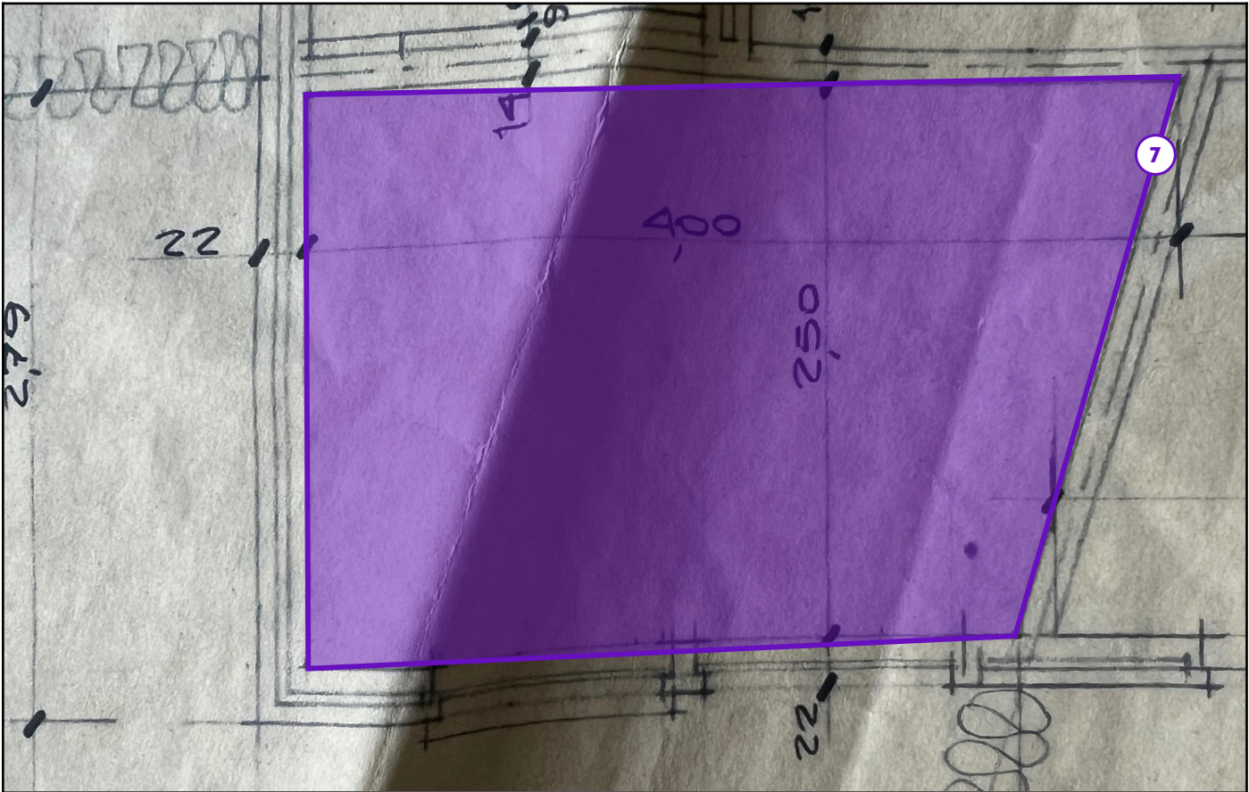
Legende van plan 2.1: Grondplan tuinhuis (baksteen)
