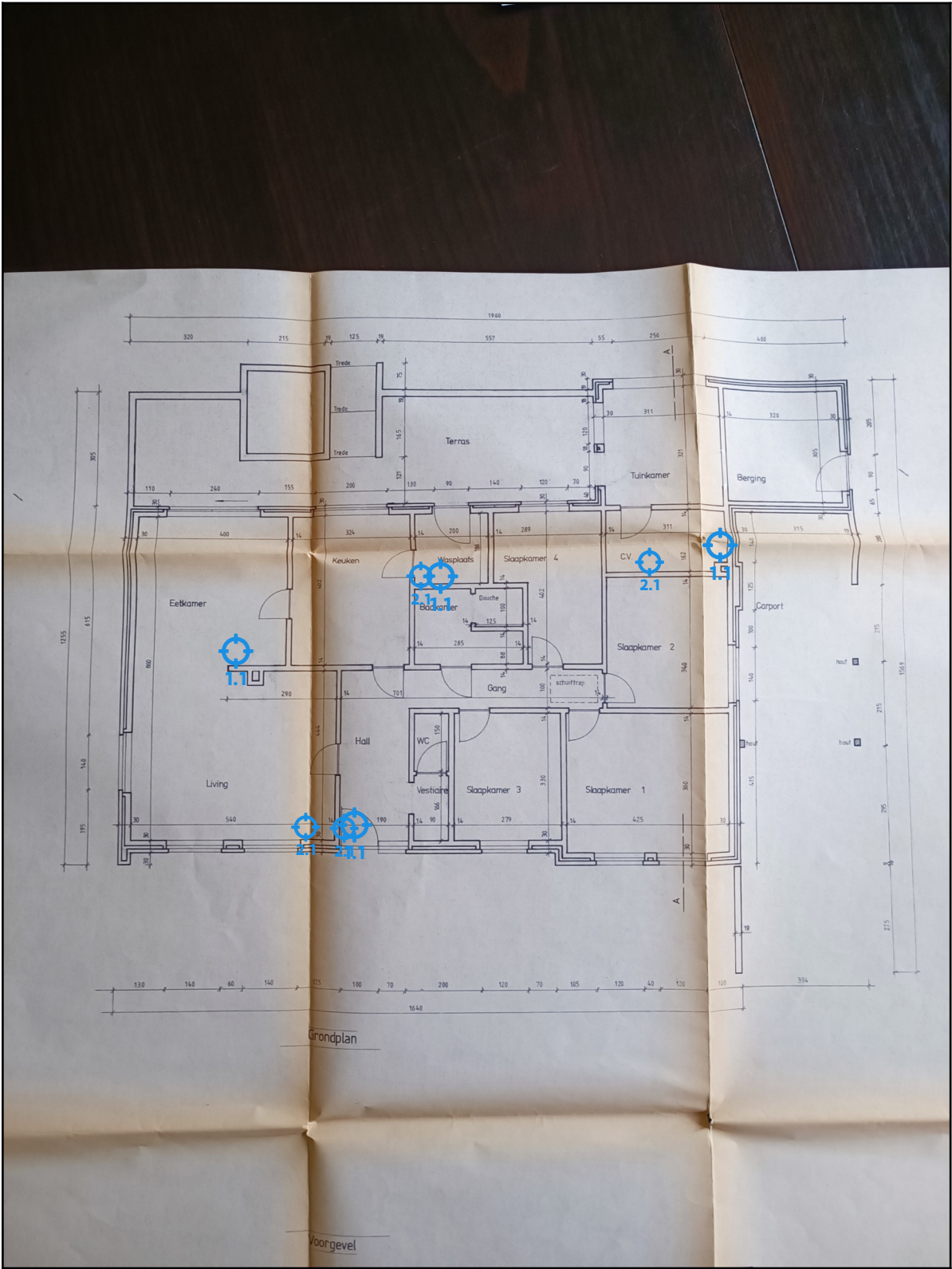
Legende van plan 1.1: grondplan gelijkvloer
