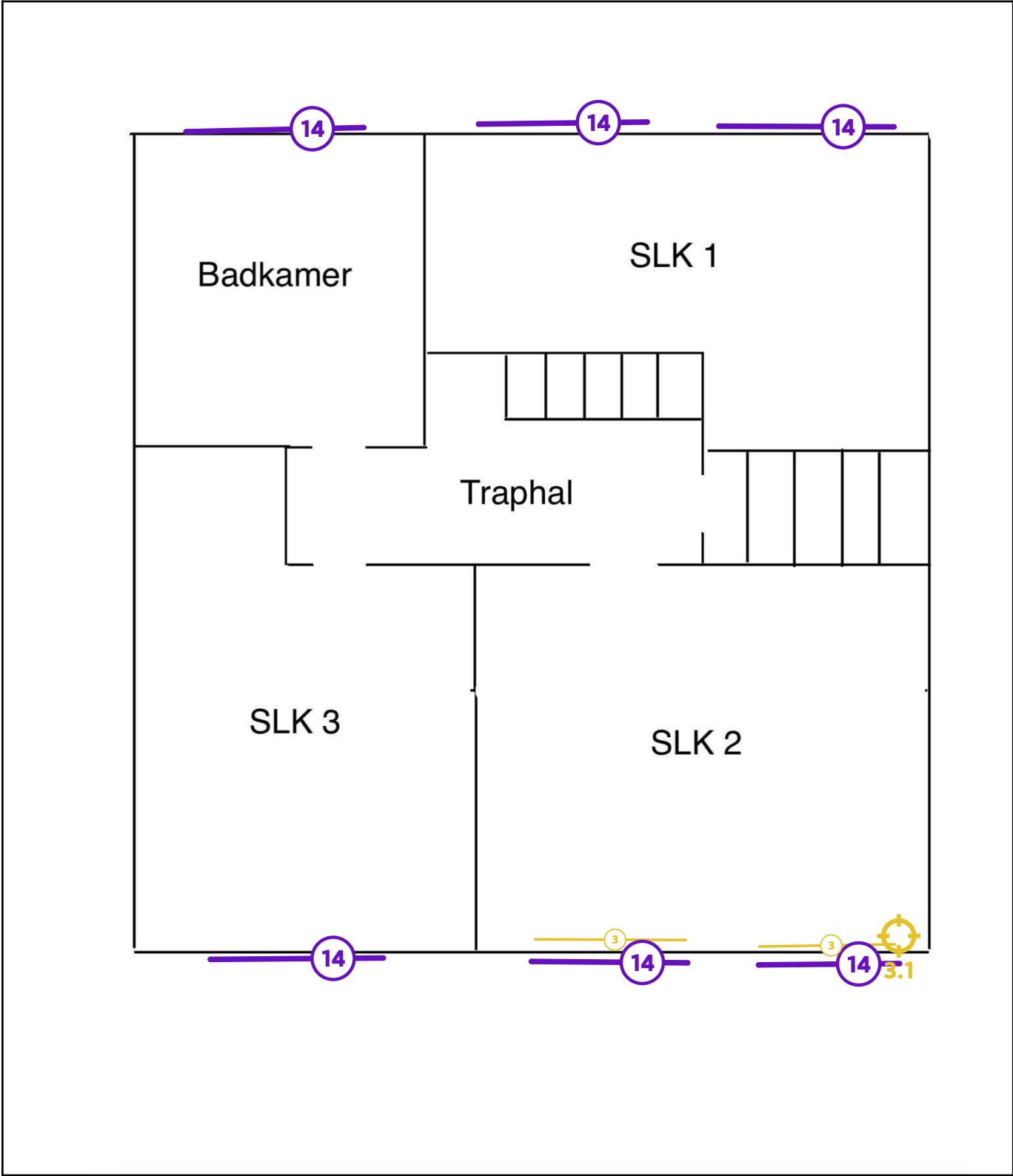
Legende van plan 1.6: Eerste verdieping
