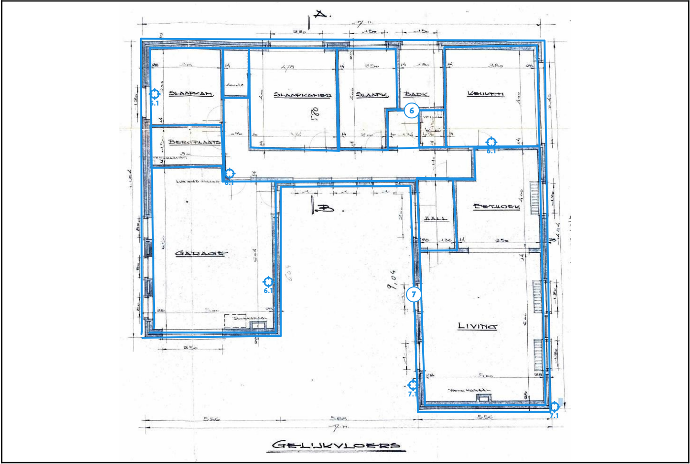
Legende van plan 1.3: Gelijkvloers (wanden)
