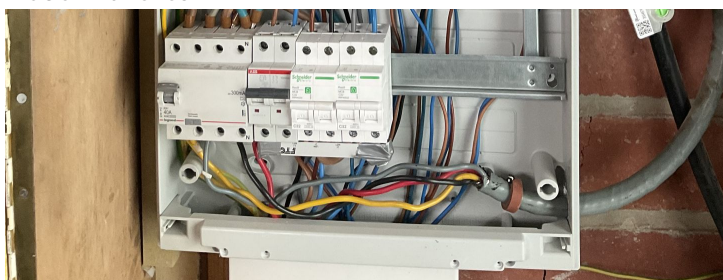
Verdeelbord 1
