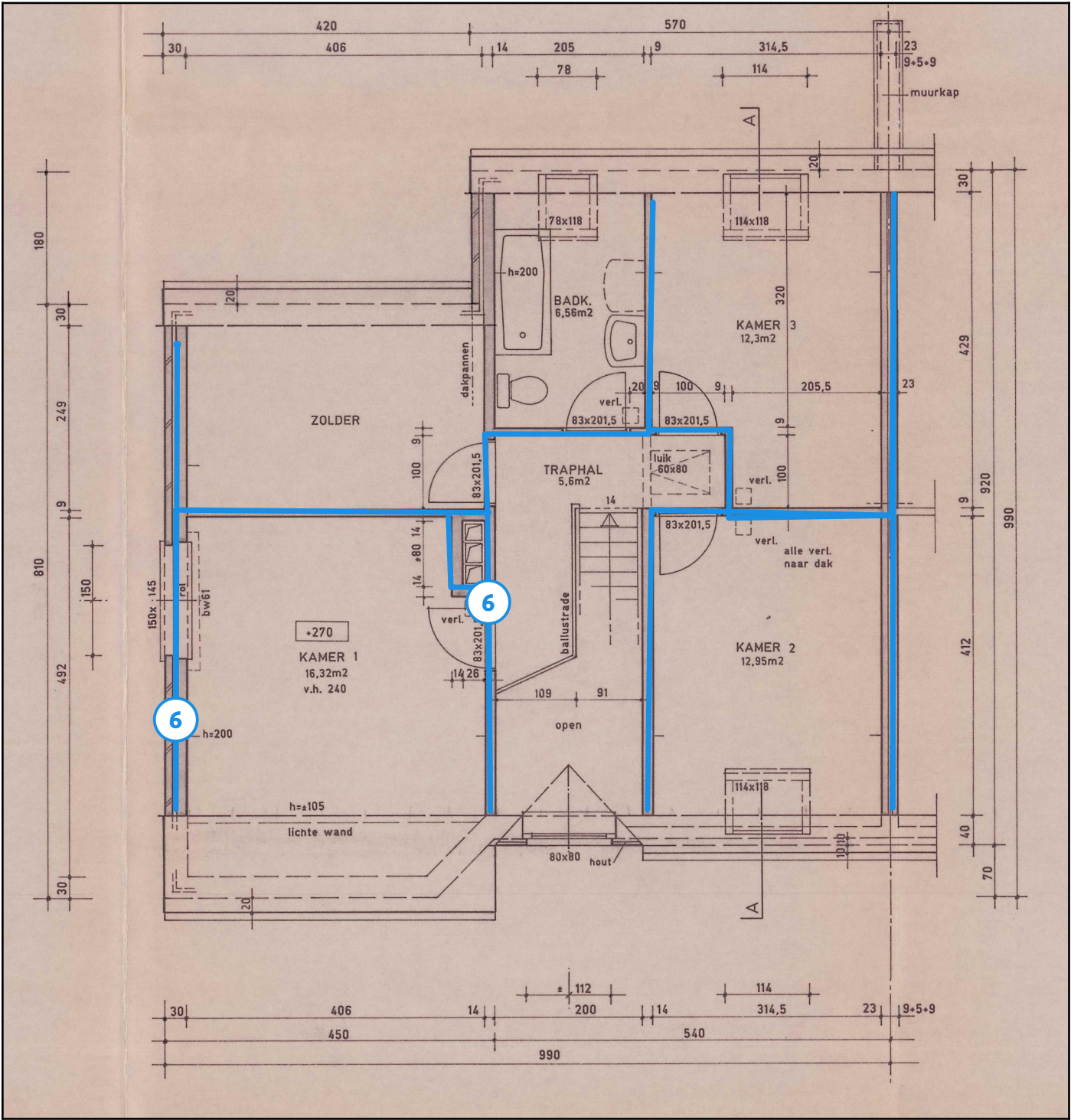
Legende van plan 1.4: Verdieping plan
