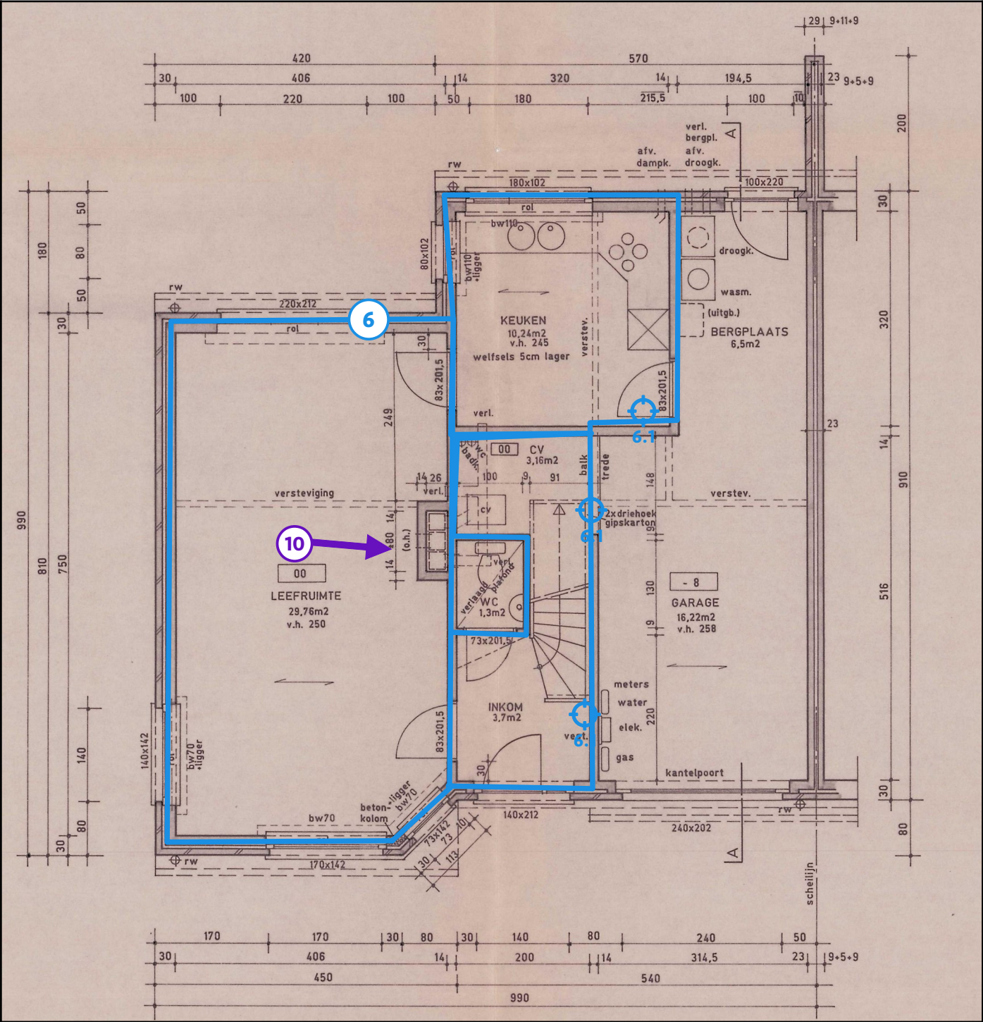
Legende van plan 1.2: Gelijkvloers plan
