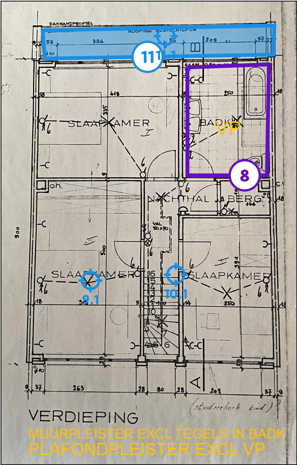
Legende van plan 1.5: Eerste verdieping
