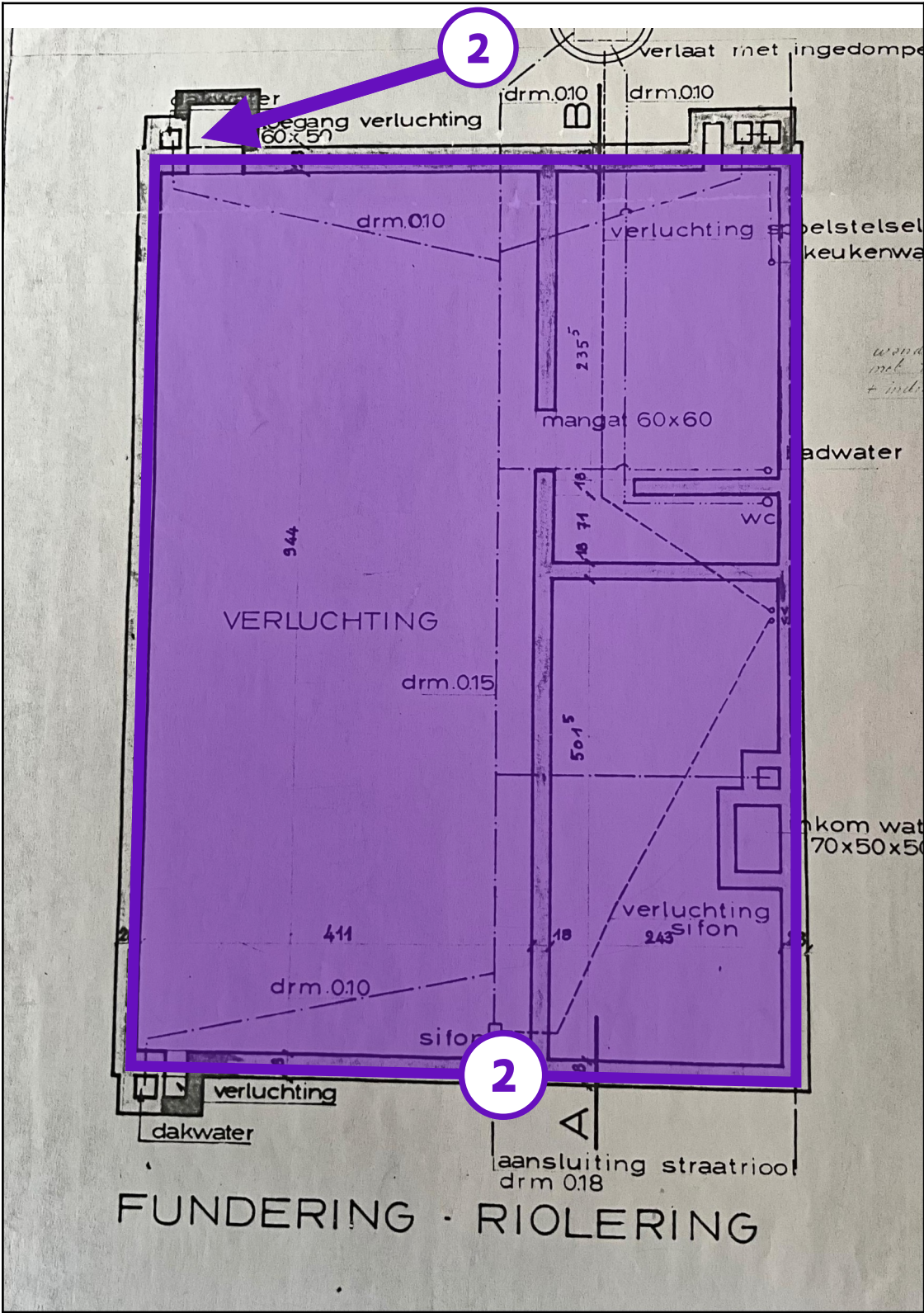
Legende van plan 1.1: Kruipruimte
