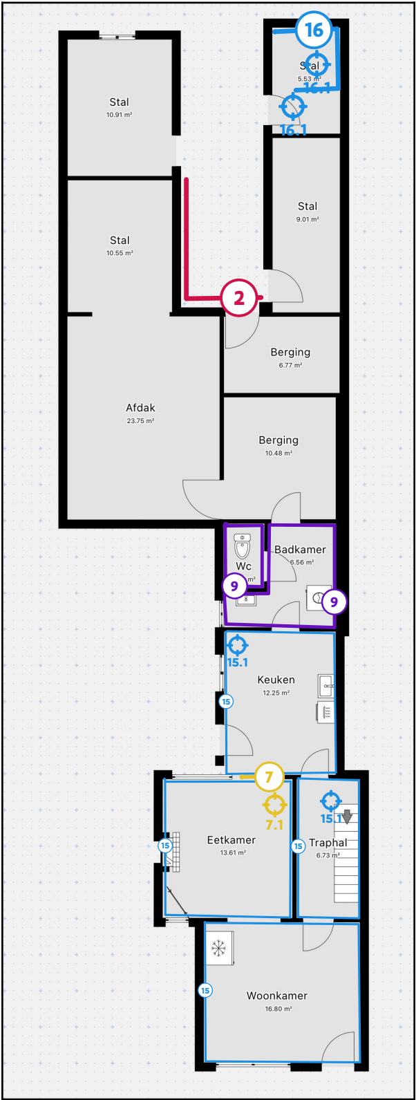
Legende van plan 1.2: Gelijkvloers - afwerking wanden
