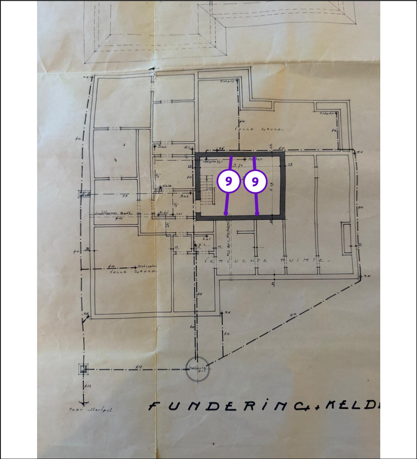
Legende van plan 1.1: Fundering- en keldering
