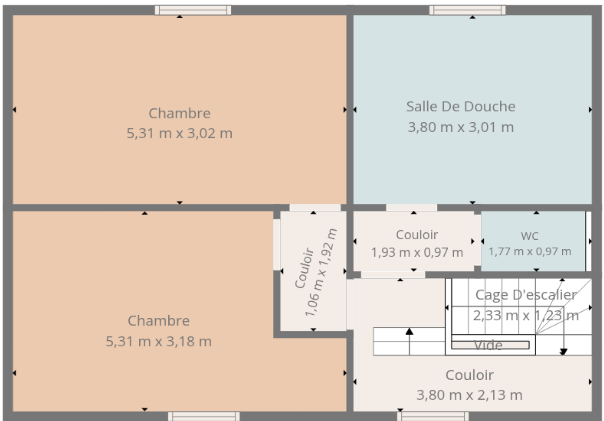
2ème Étage
