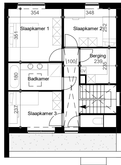
NIVEAU +1 1/150
