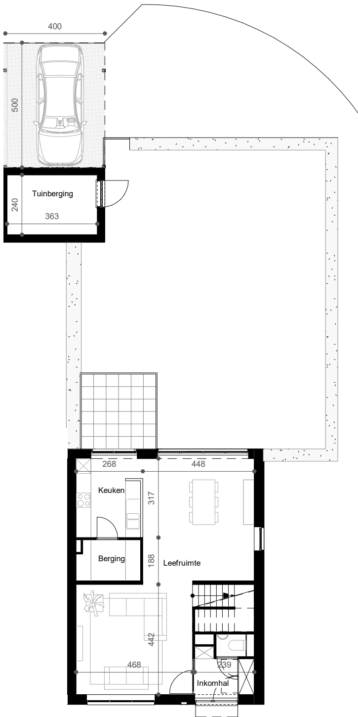
NIVEAU +0 1/150
