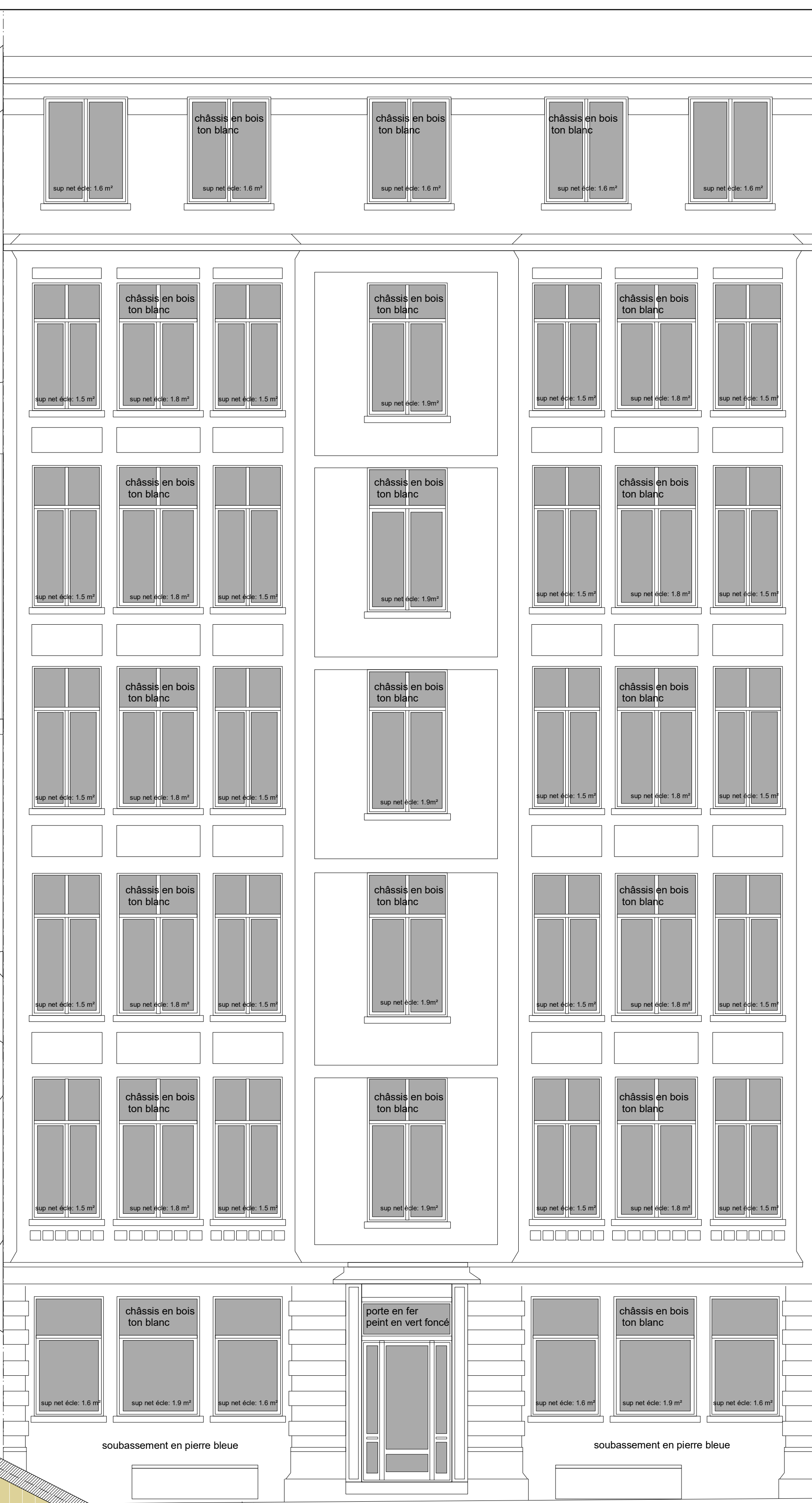
FACADE AVANT
