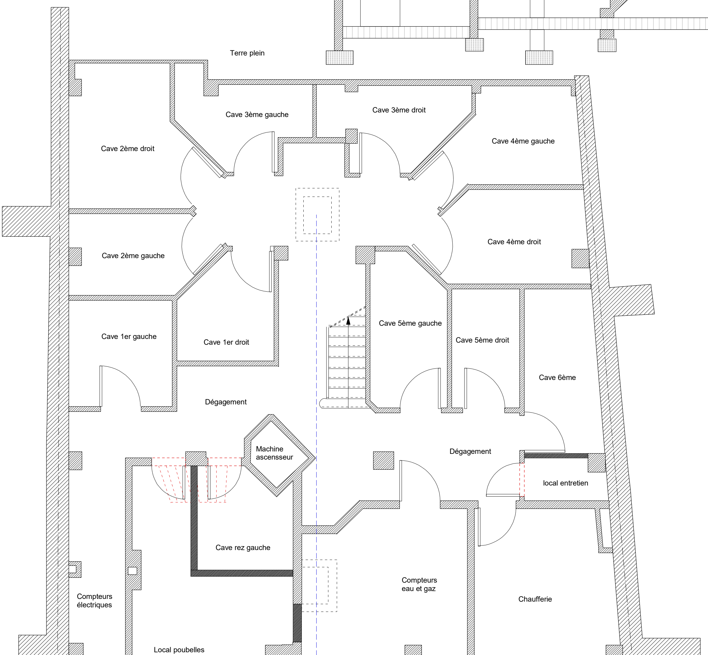
PLAN SOUS-SOL
