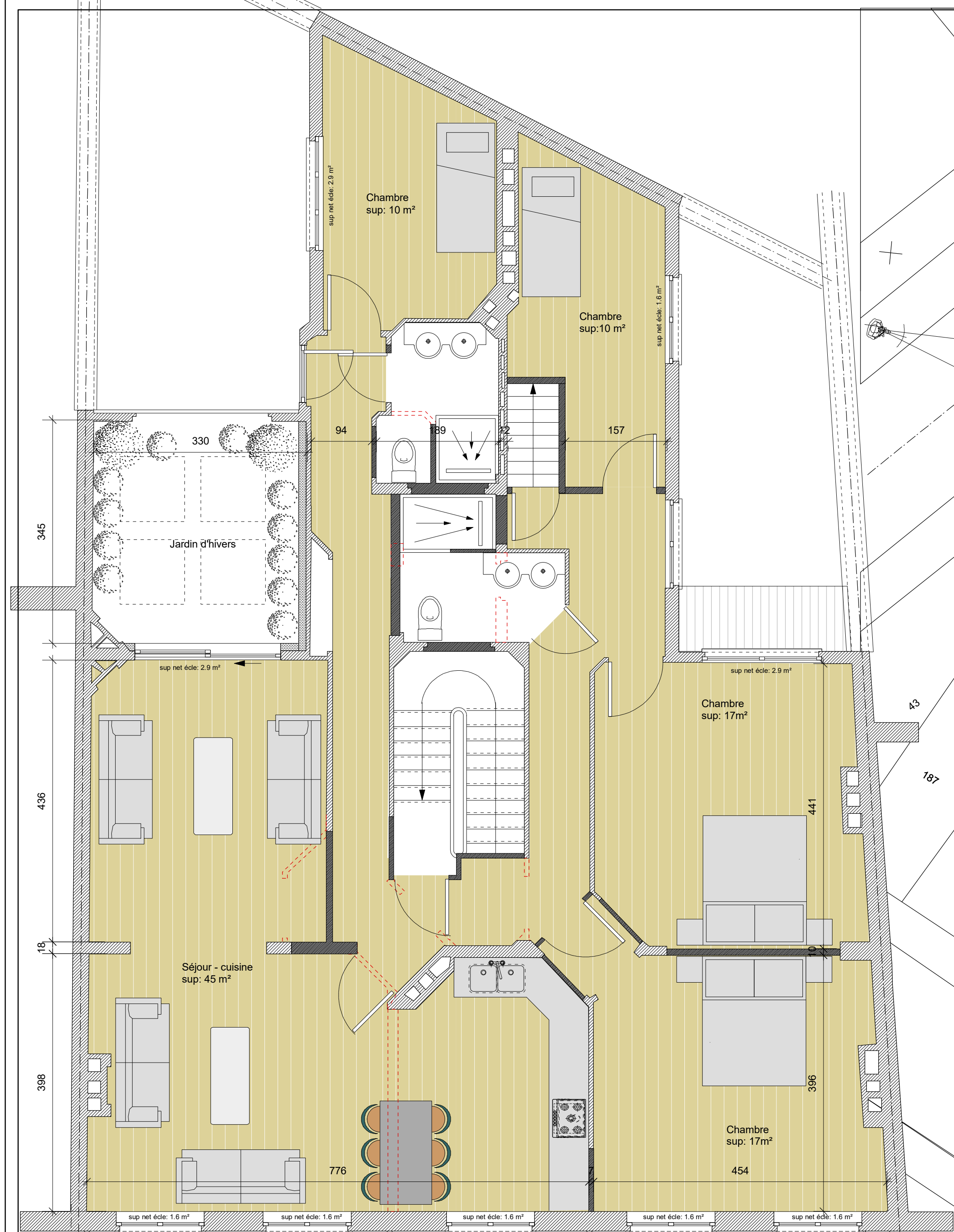
PLAN 6ème ETAGE
