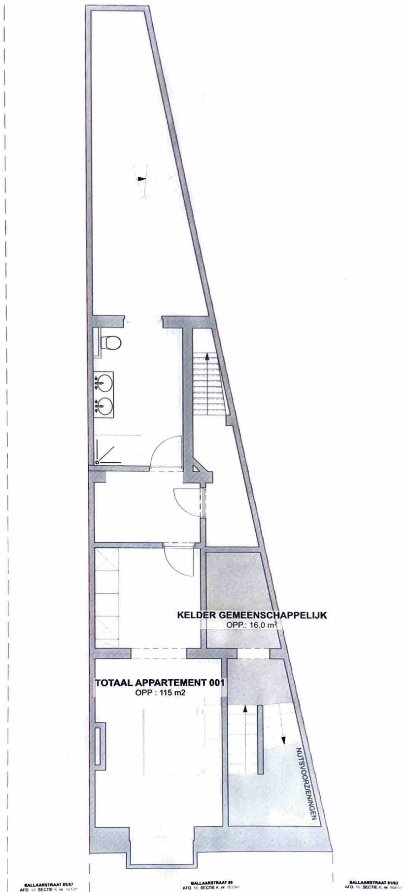
GRONDPLAN NIVEAU -0.5 APPARTEMENT 001, DUPLEX NIEUWE TOESTAND
