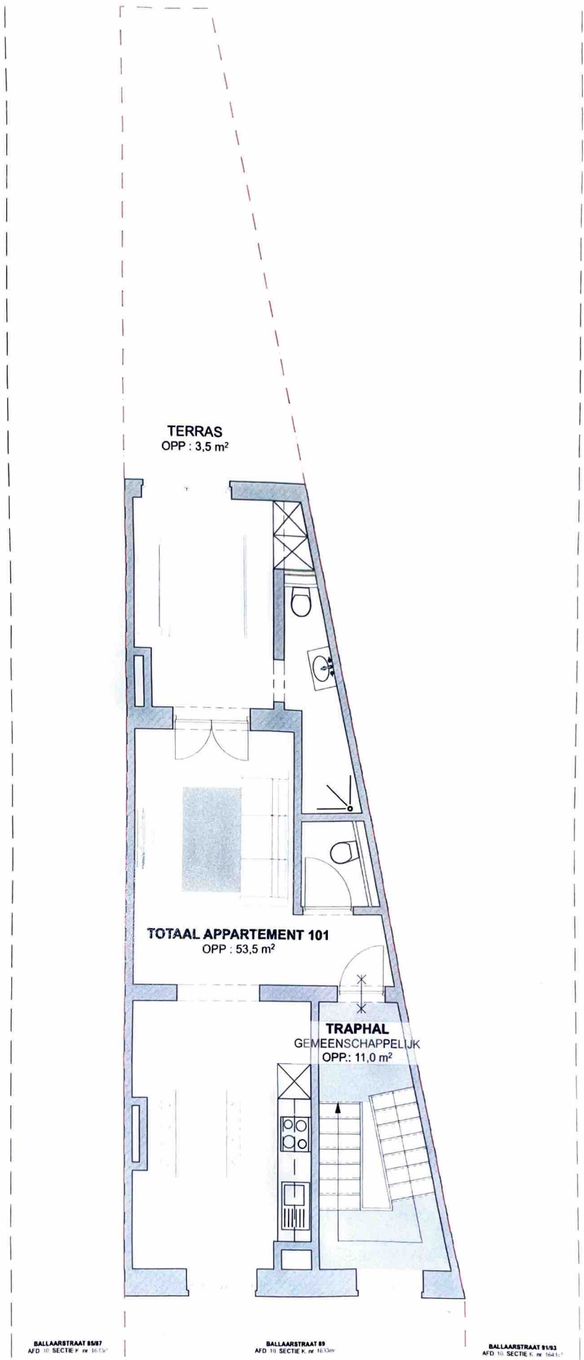
GRONDPLAN NIVEAU +1 APPARTEMENT 101 NIEUWE TOESTAND
