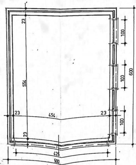
grondplan
