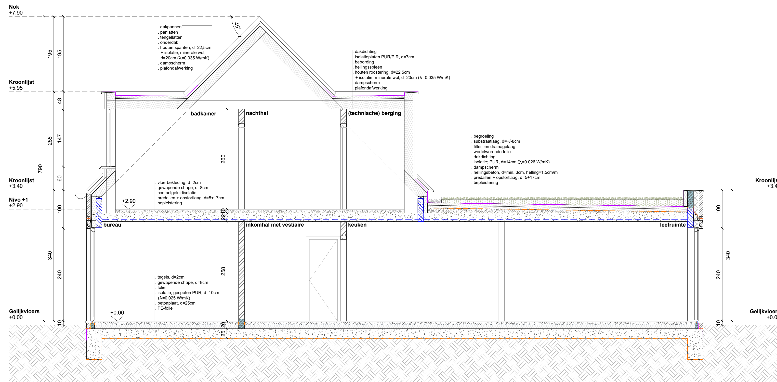
SNEDE
