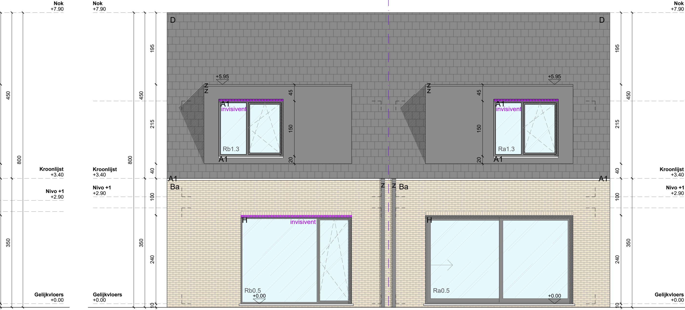
ACHTERGEVEL
