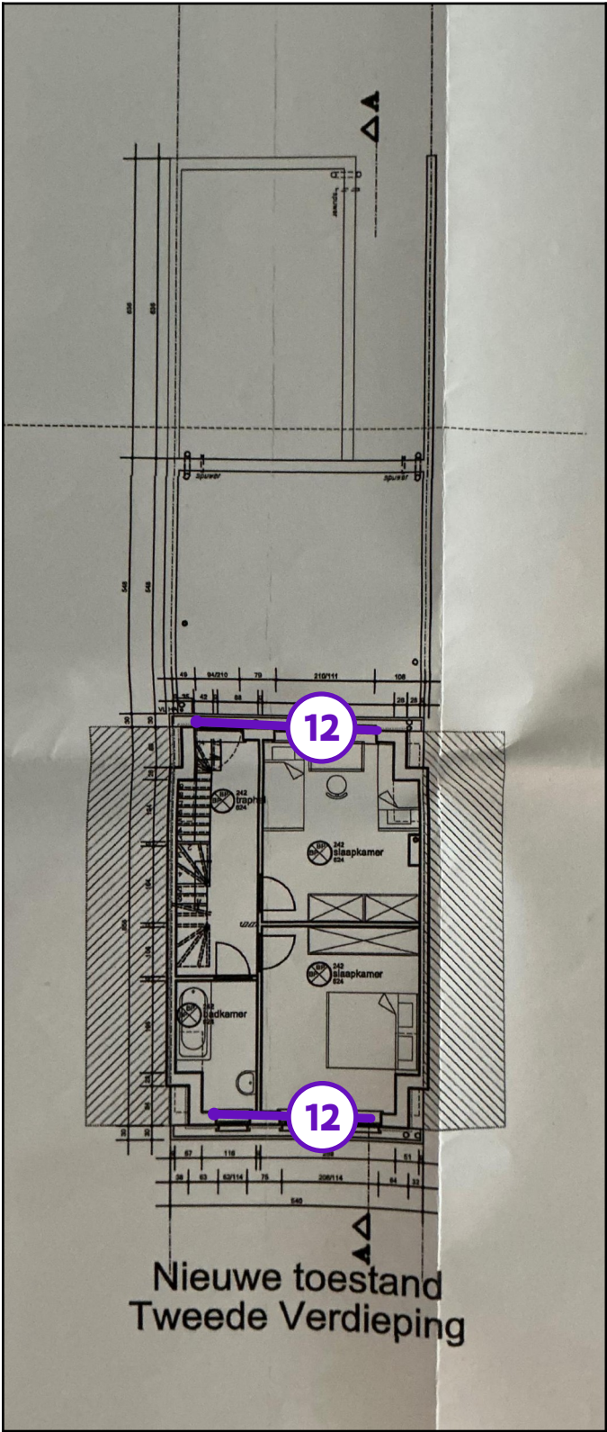
Legende van plan 1.8: Tweede verdiep
